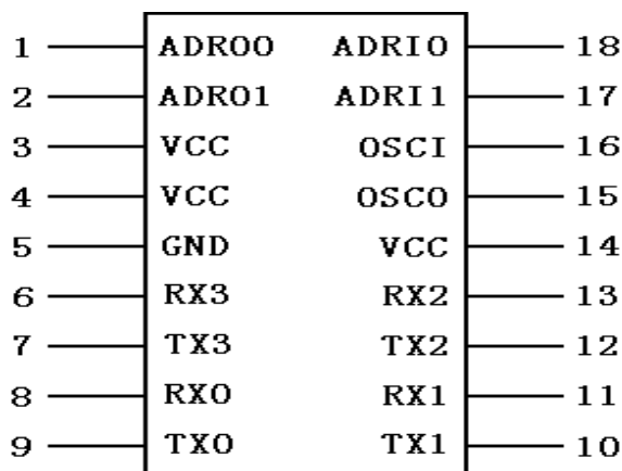
图 1 DIP 和 SOIC 封装
