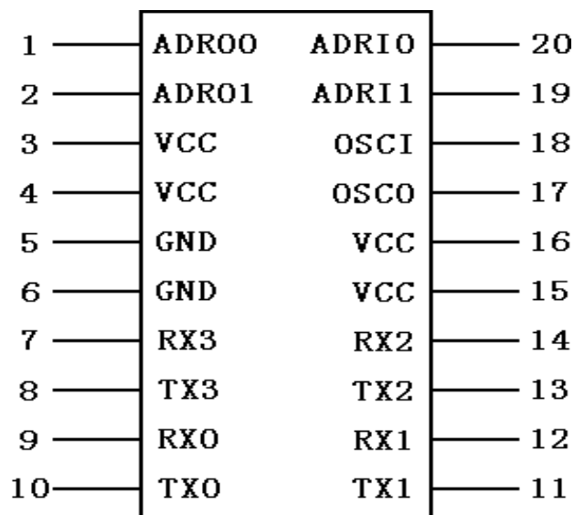
图2 SSOP封装
