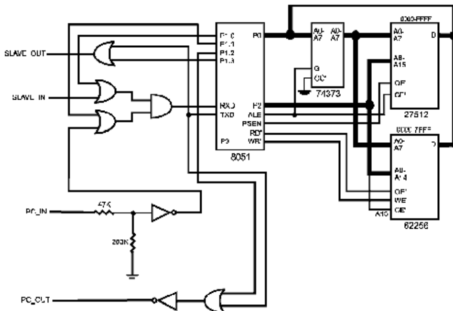
图0-1 复用串行端口
