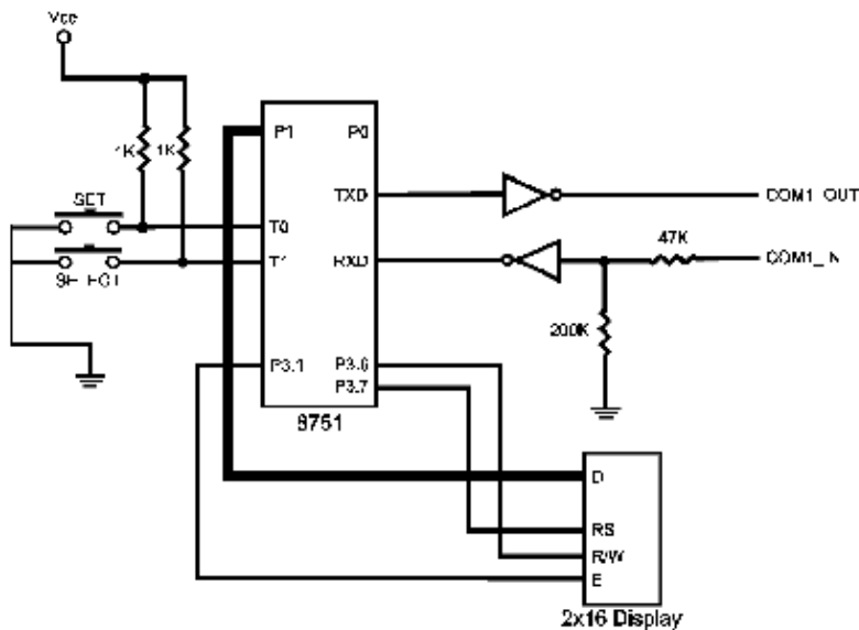
图0-3 时钟作为从设备
