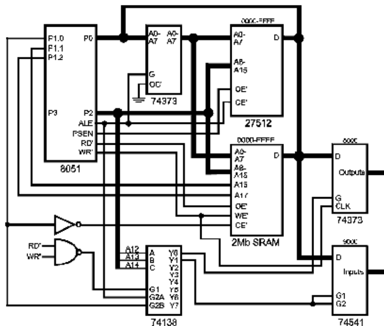
图0-4 页寻址RAM
