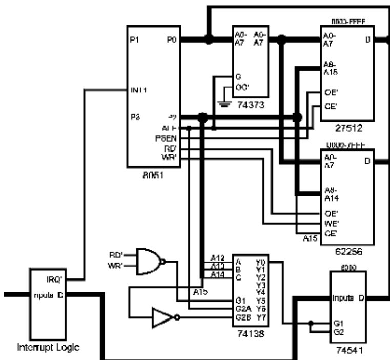
图0-2 共享外部中断
