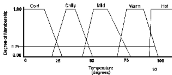
图0-1 温度函数
