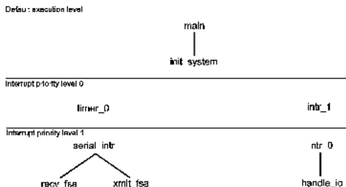
图0-1 简单调用树
