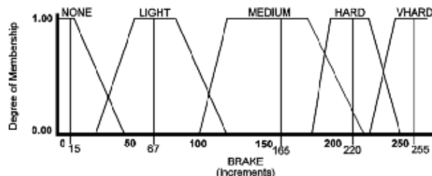
图0-9 输出功能函数
