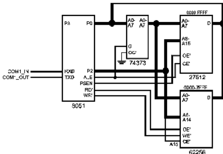
图 0-6 8051作为高速从器件
