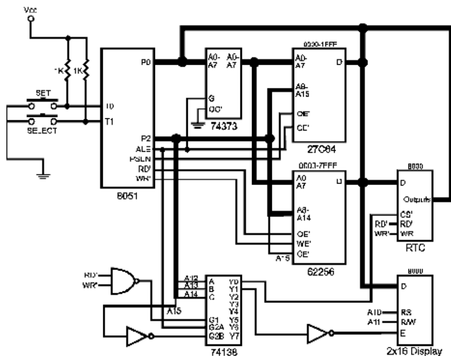
图 0-2 扩展电路
