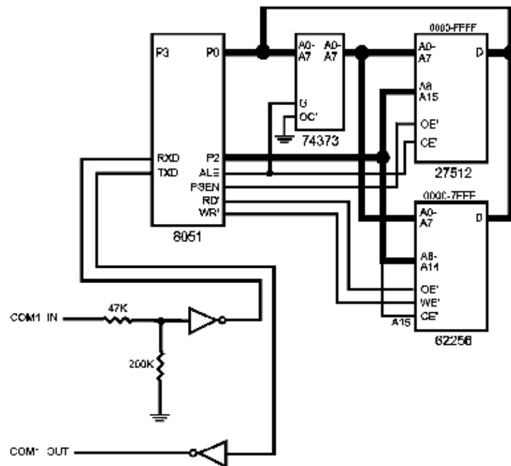
图0-1 PC接口
