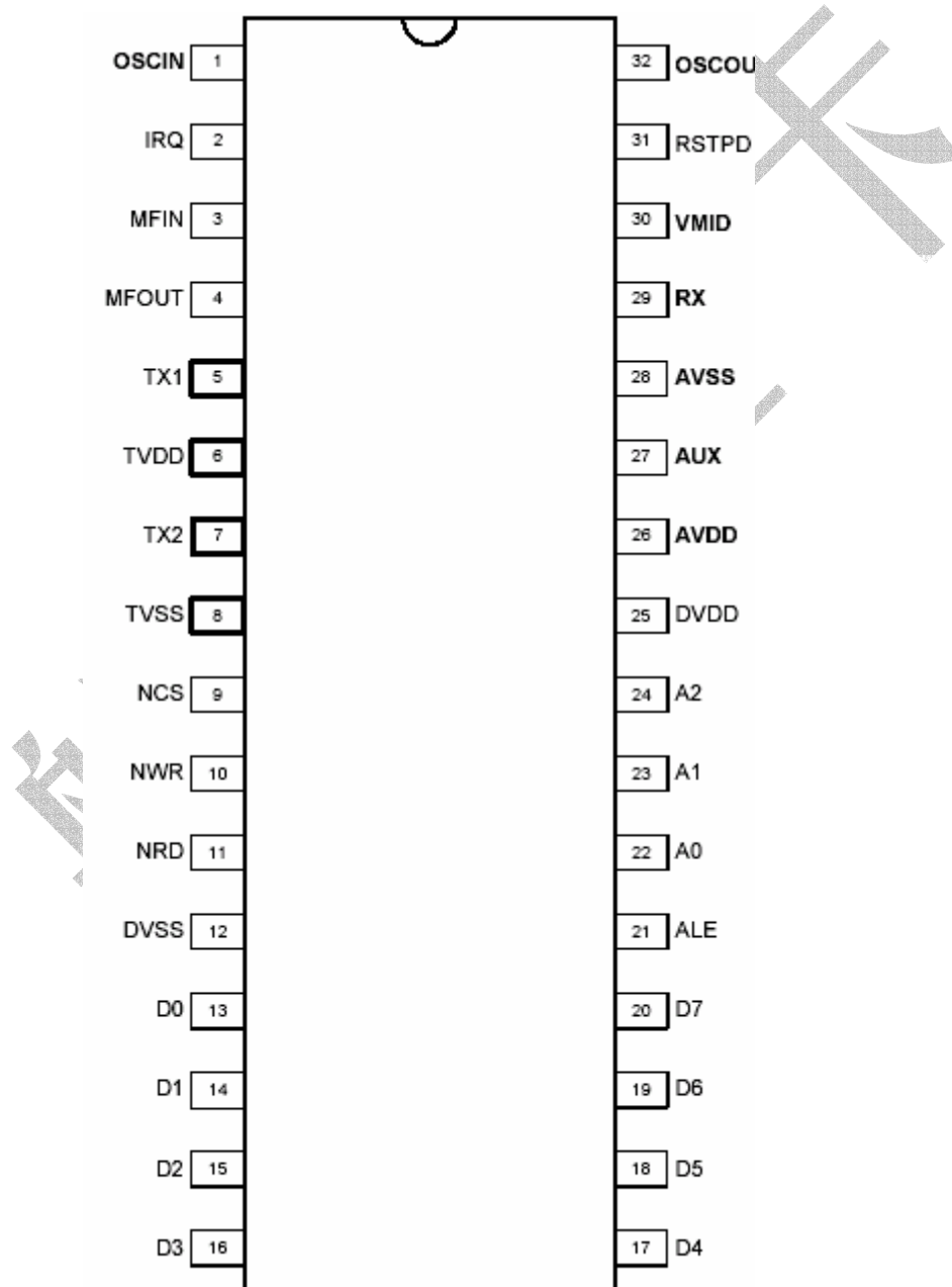
图 3 - 1 : FM1702/1704/1705 管脚配置 ( SOP32 封装 )
