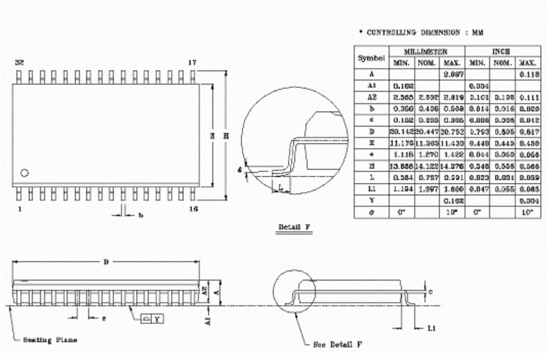
图 23 - 1 : SOP32 封装
