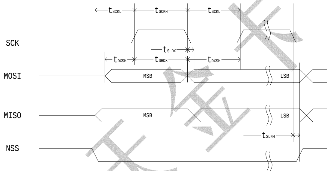
图 20 - 4：SPI 时序图
