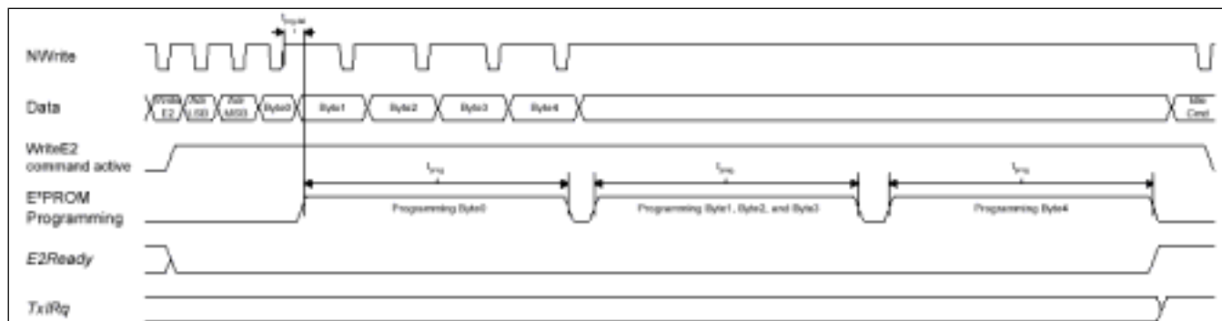
图 16 - 5：E²PROM 编程的时序图
