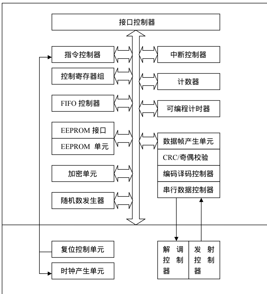
图 2 - 1 : FM1702/1704/1705 结构图
