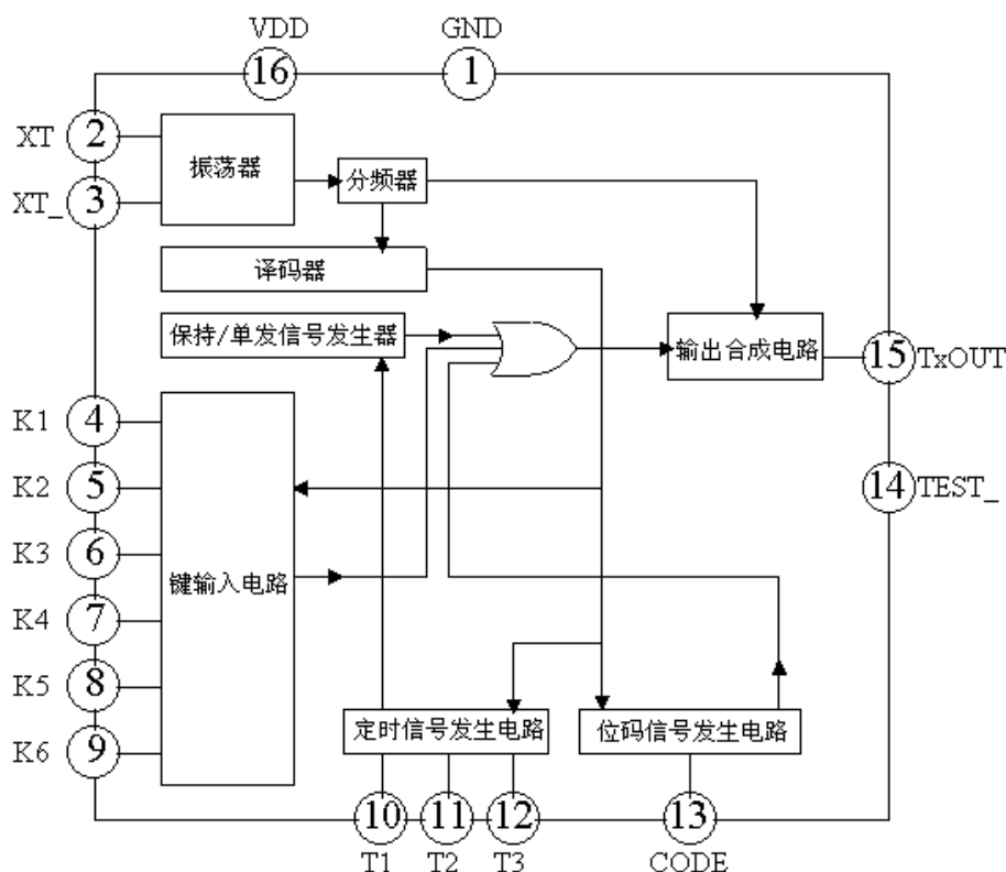
管脚图
