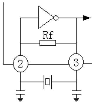
晶振电路
