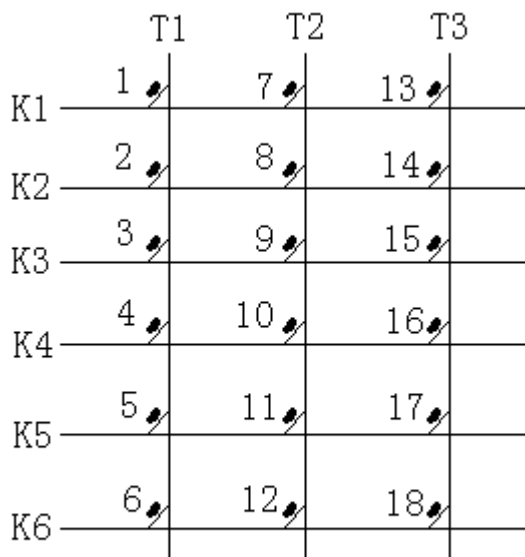
9148 键盘矩阵
