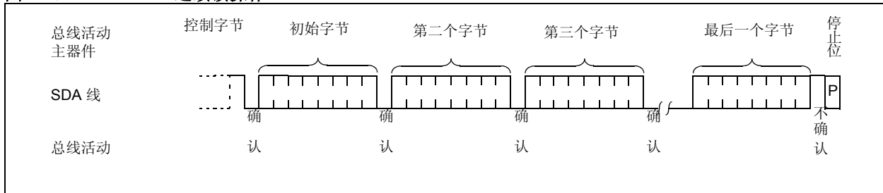
图 8-4: 连续读操作
