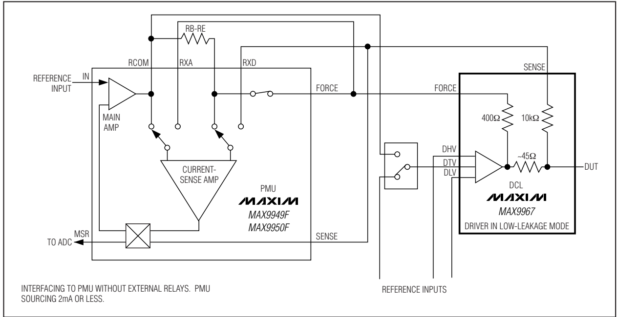
典型应用电路 (简图)
