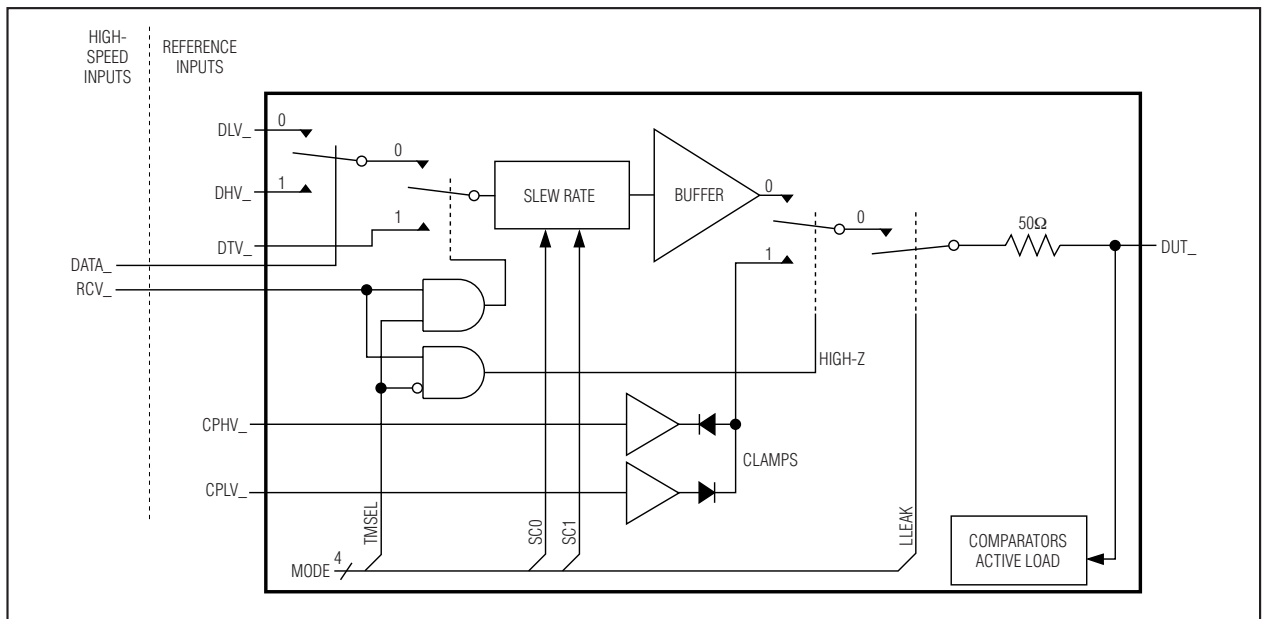
图2. 简化驱动器通道
