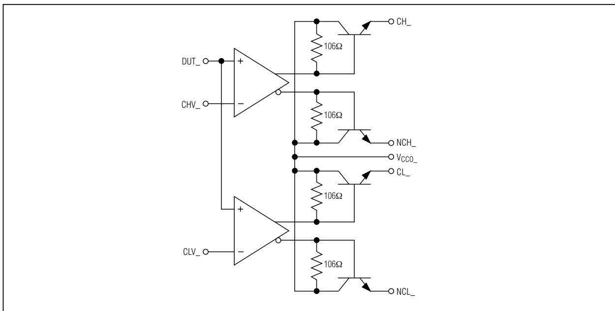
图4. 比较器射极开路输出
