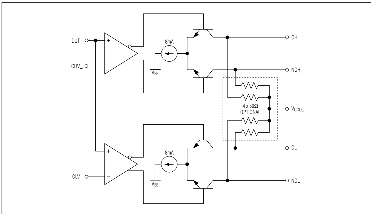
图3. 比较器集电极开路输出
