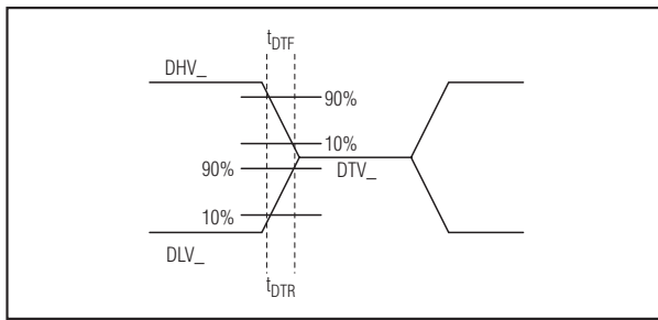
图 1a. 驱动至终端的上升和下降时间
