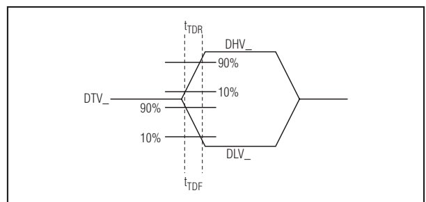
图 1b. 终端至驱动的上升和下降时间
