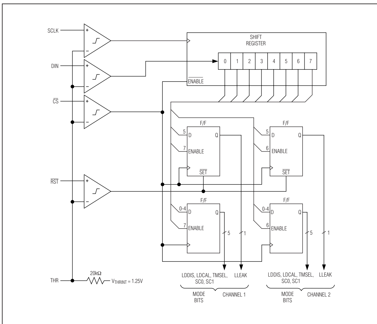
图5. 串行接口
