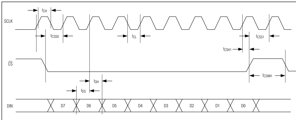
图6. 串口时序
