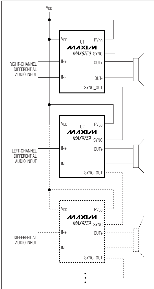
图7. 主从式配置方案
