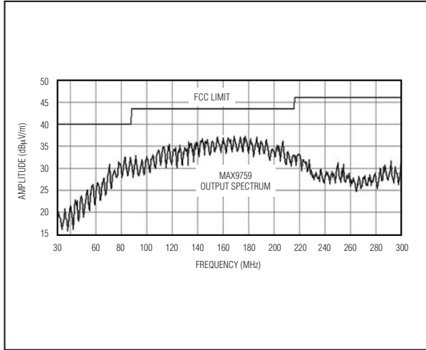
图3. MAX9759的EMI频谱
