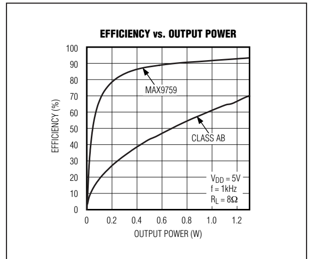
图5. MAX9759效率与输出功率的关系
