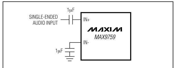
图6. 单端输入
