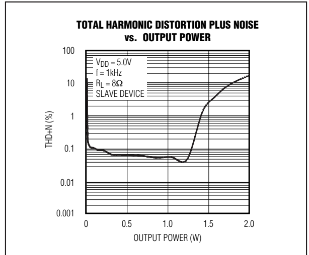
图8. 总谐波失真+噪声与输出功率的关系
