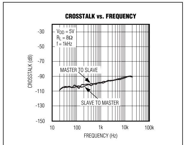
图9. 串扰与频率的关系
