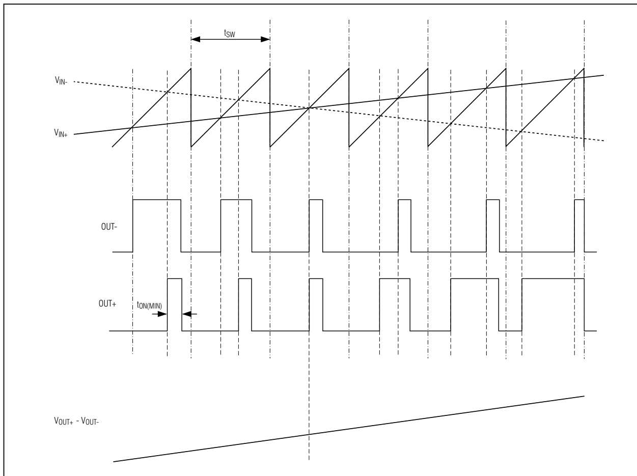
图1. MAX9759加载输入信号时的输出波形
