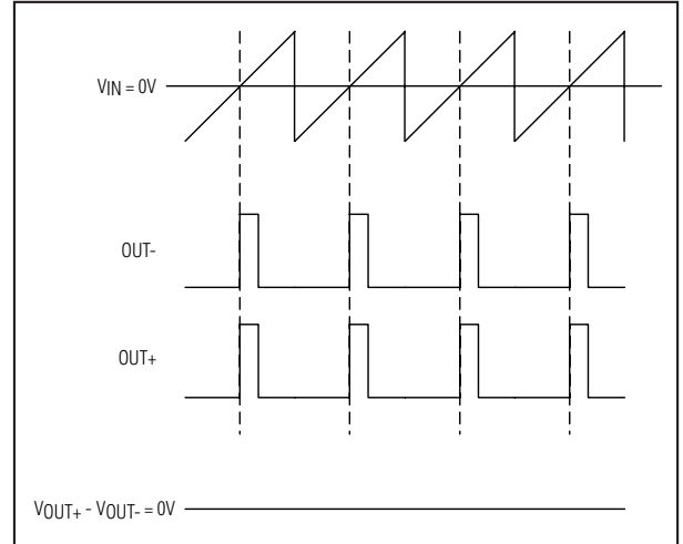
图4. 无输入信号时MAX9759的输出波形
