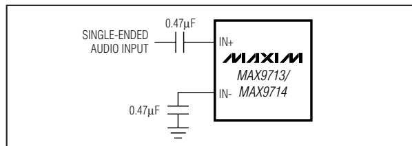
图 5. 单端输入
