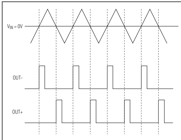
图1. 无输入信号时MAX9714的输出
