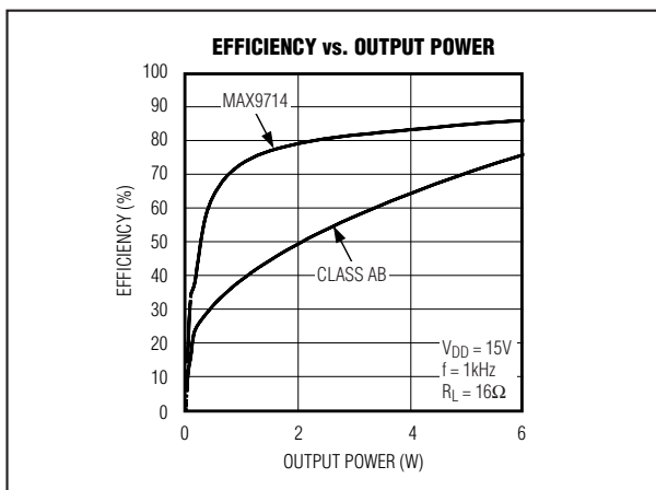
图 3. MAX9714 效率与 AB 类效率对比
