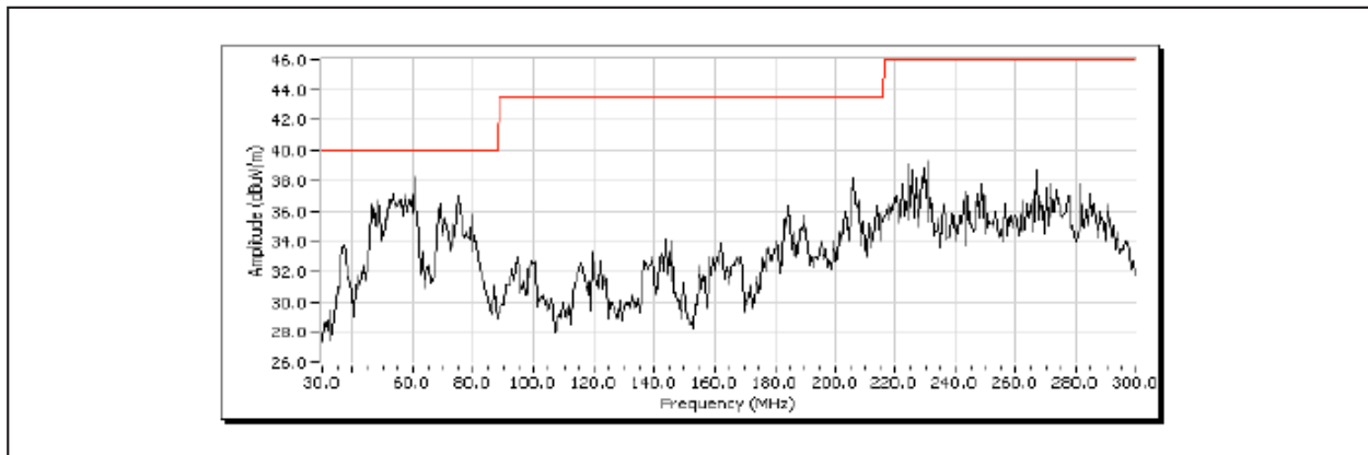
图 2. SSM 辐射
