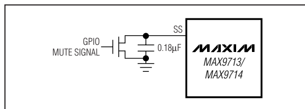
图 4. MAX9713/MAX9714 静音电路
