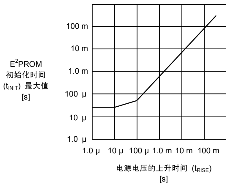
图 27 E 2 PROM 的初始化时间
