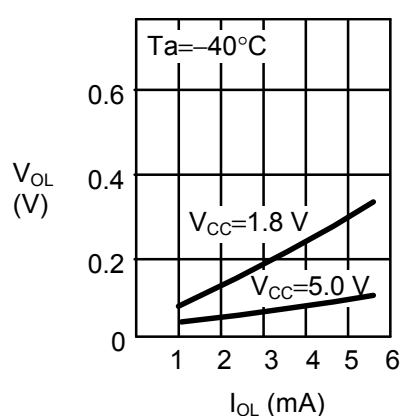
1.18 低电平输出电压( V_{OL} ) — 低电平输出电流( I_{OL} )
