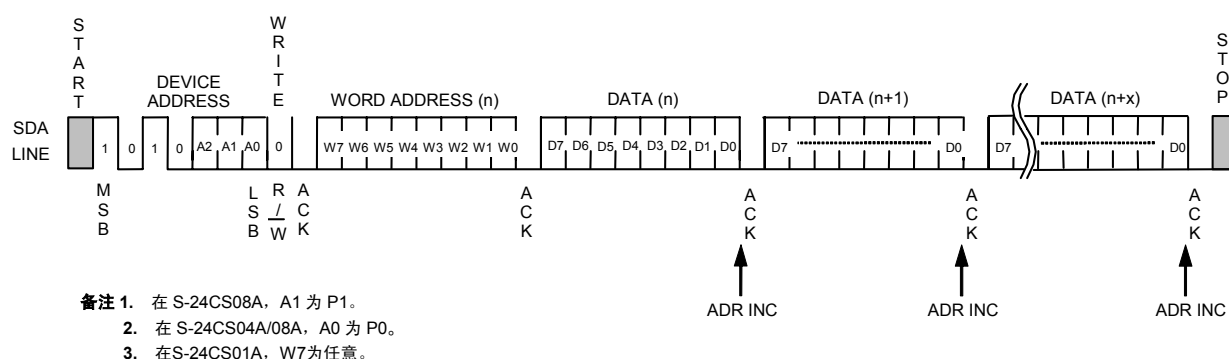
图14 页写入
