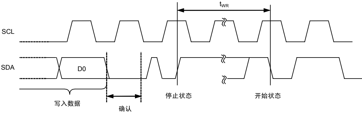
图8 写入周期定时
