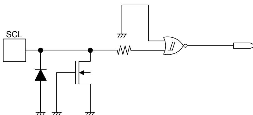
图 21 SCL 端子
