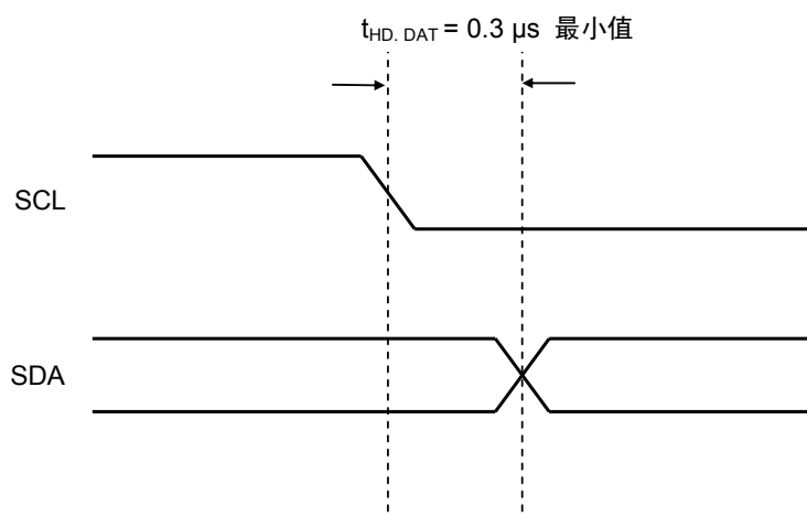
图 28 E 2 PROM 的数据保持时间
