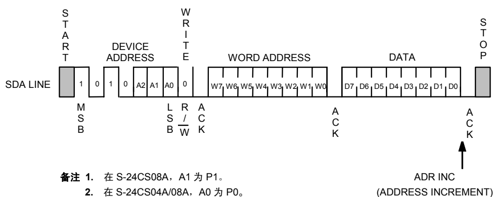
图13 字节写入
