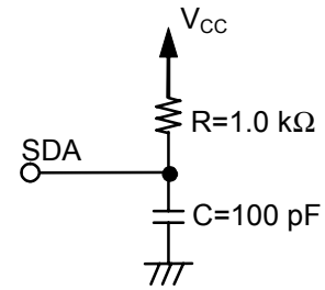
图6 输出负载电路
