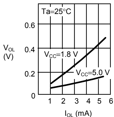
1.17 低电平输出电压( V_{OL} ) — 低电平输出电流( I_{OL} )
