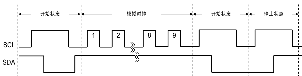
图24 E 2 PROM的复位方法
