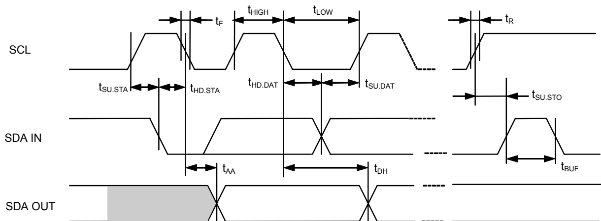
图7 总线定时
