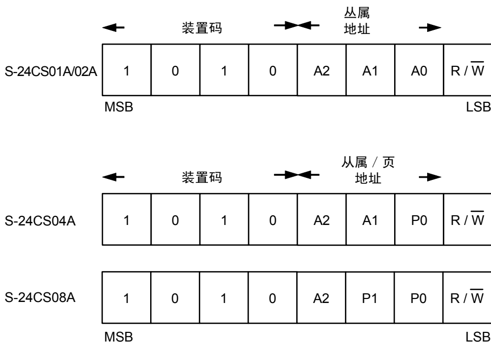
图12 装置地址
