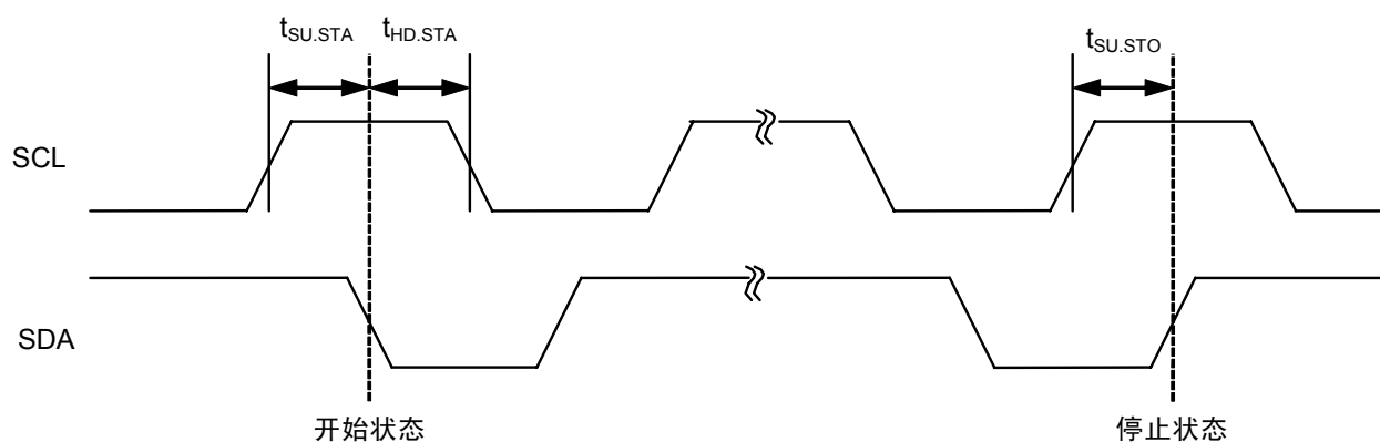
图9 开始/停止状态
