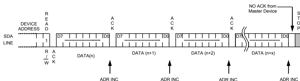
图17 顺序读出
