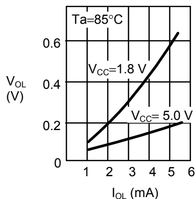
1.18 低电平输出电压( V_{OL} ) — 低电平输出电流( I_{OL} )
