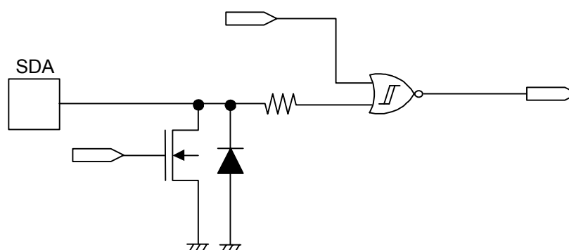
图 22 SDA 端子
