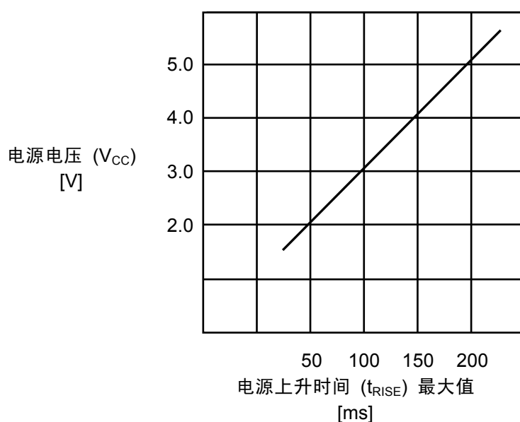
图 26 电源电压上升时间
