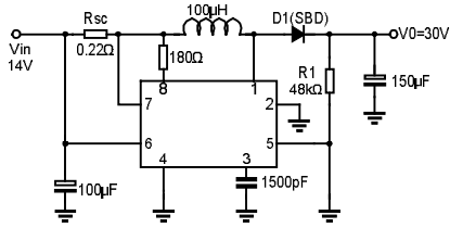
图1 升压变换器
