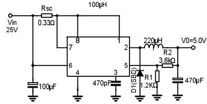
图2 降压变换
