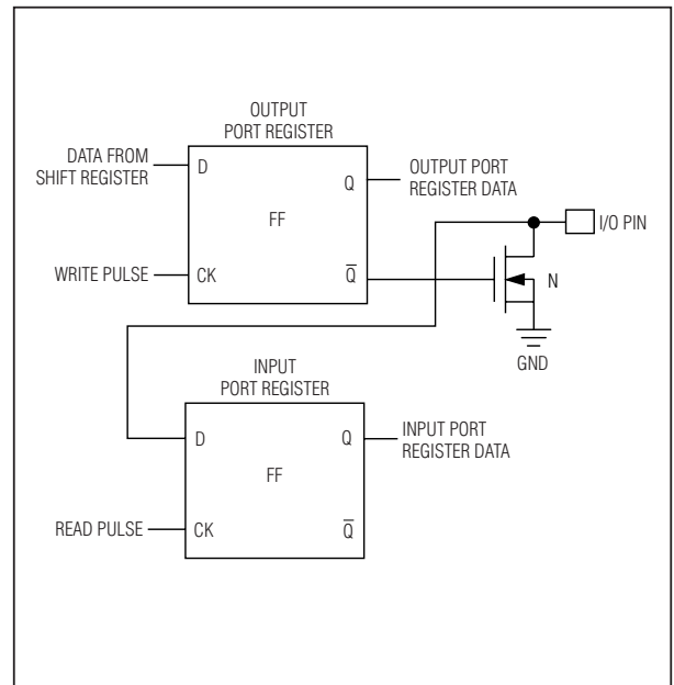
图 1. I/O 端口的简化原理图
