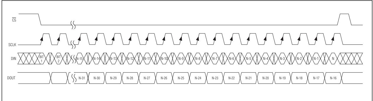
图 6. 向 MAX7317 发送超过 16 位数据
