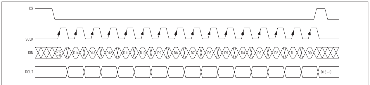
图 5. 16 位写操作发送至 MAX7317
