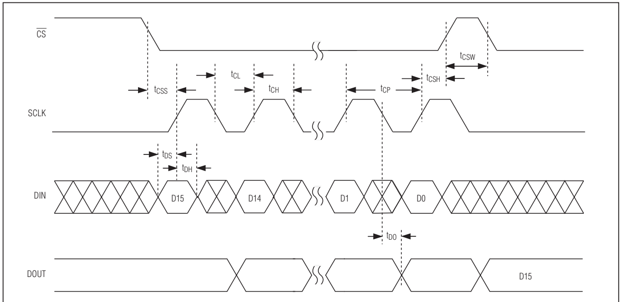
图 4. 时序图
