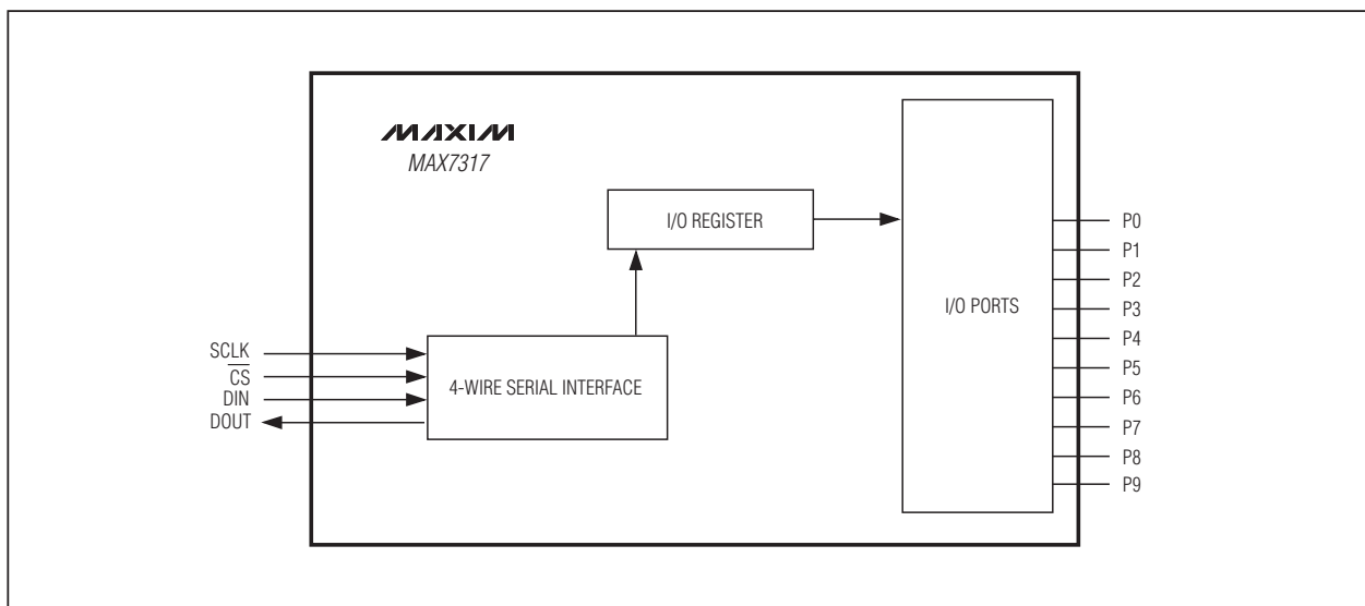
MAX7317 方框图
