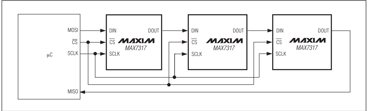
图 3. MAX7317 菊花链连接
