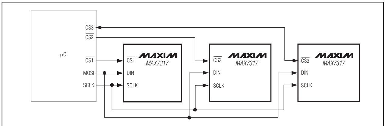
图 2. MAX7317 多 \overline{CS} 线连接
