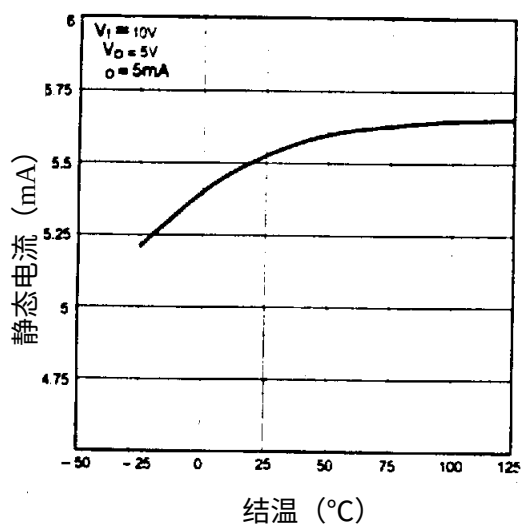
静态电流
