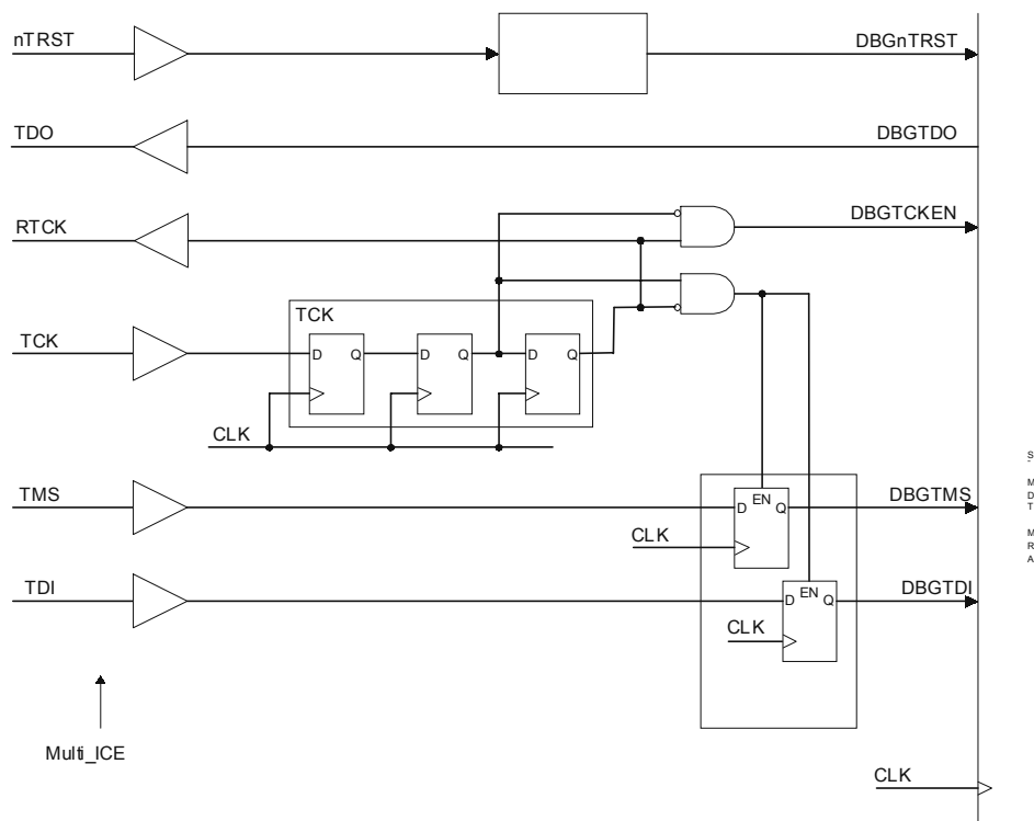
图 5-4 时钟同步
