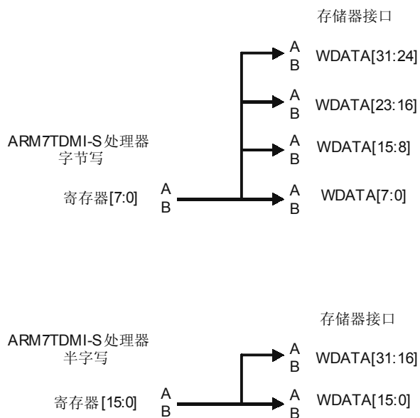
图 3-6 数据复制
