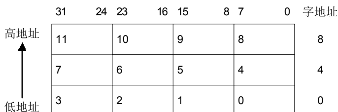
图 2-2 字内字节的小端地址
