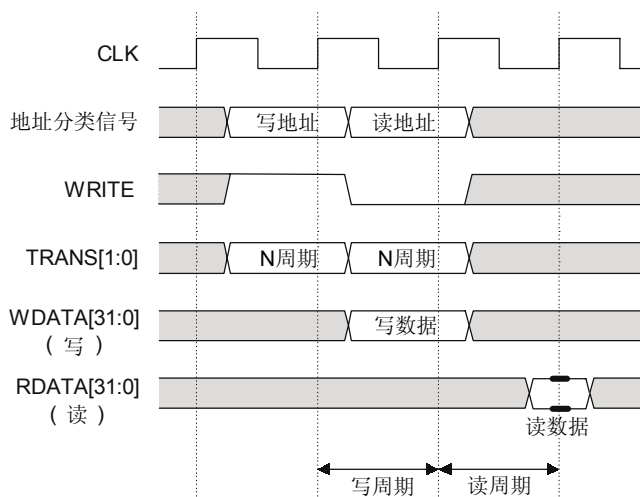
图 3-3 背靠背 的存储器周期
