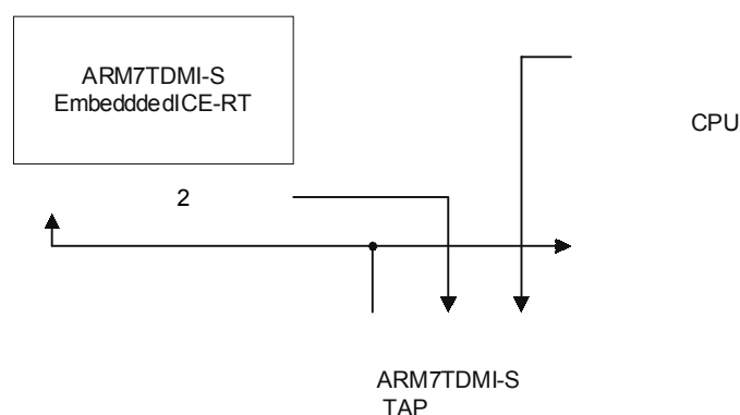
图 5-7 ARM7TDMI-S 扫描链排列
