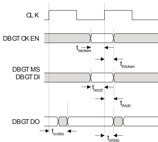
图 8-5 扫描时序
