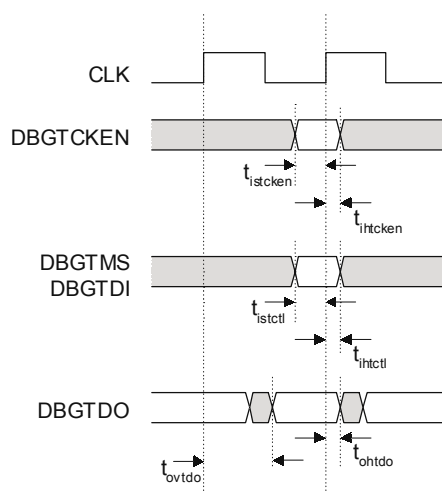
图 5-10 扫描时序
