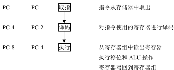
图 1-1 指令流水线
