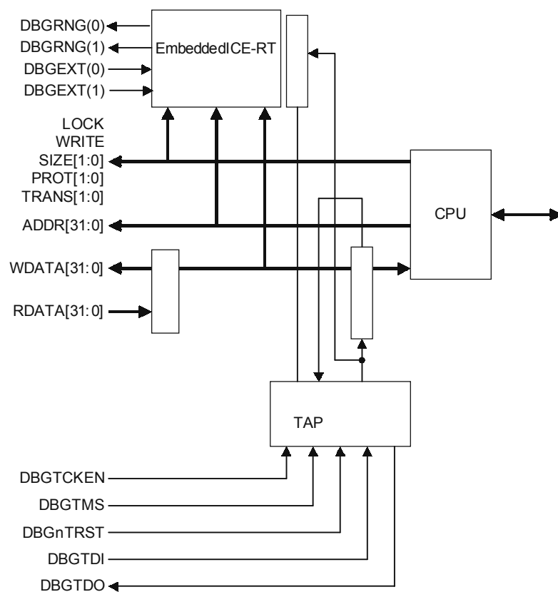
图 1-2 ARM7TDMI-S 模块
