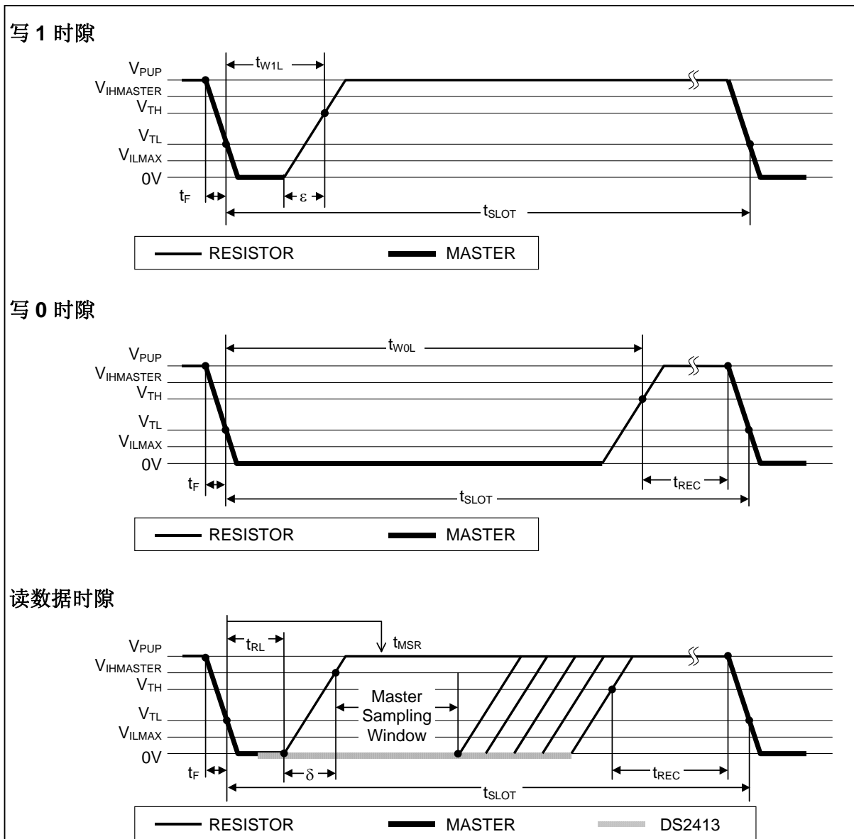
图 12. 读/写时隙图
