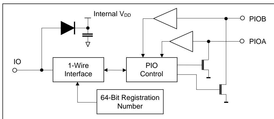
图 1. 内部框图
