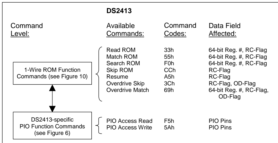
图 2. 1-Wire 协议的层次结构
