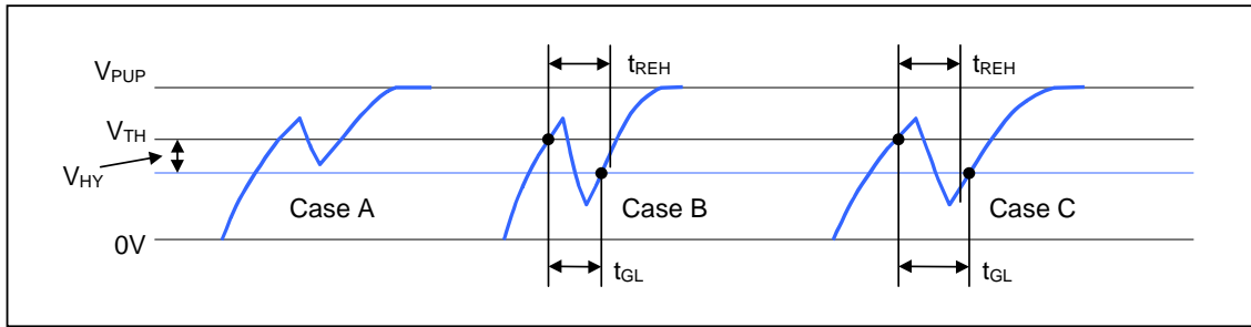
图 13. 噪声抑制示意图
