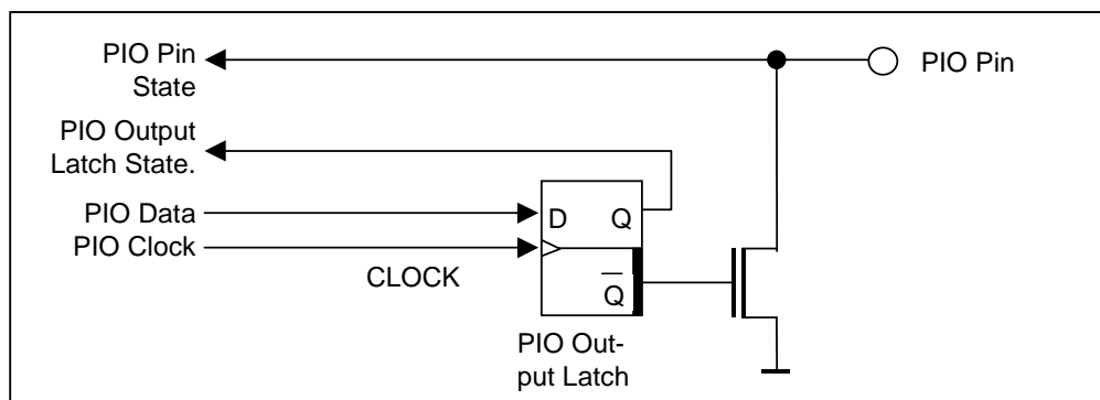
图 5. PIO 简化逻辑框图
