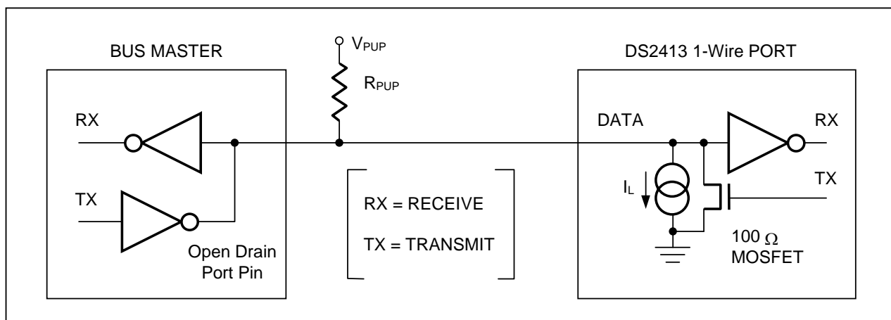
图 9. 硬件配置
