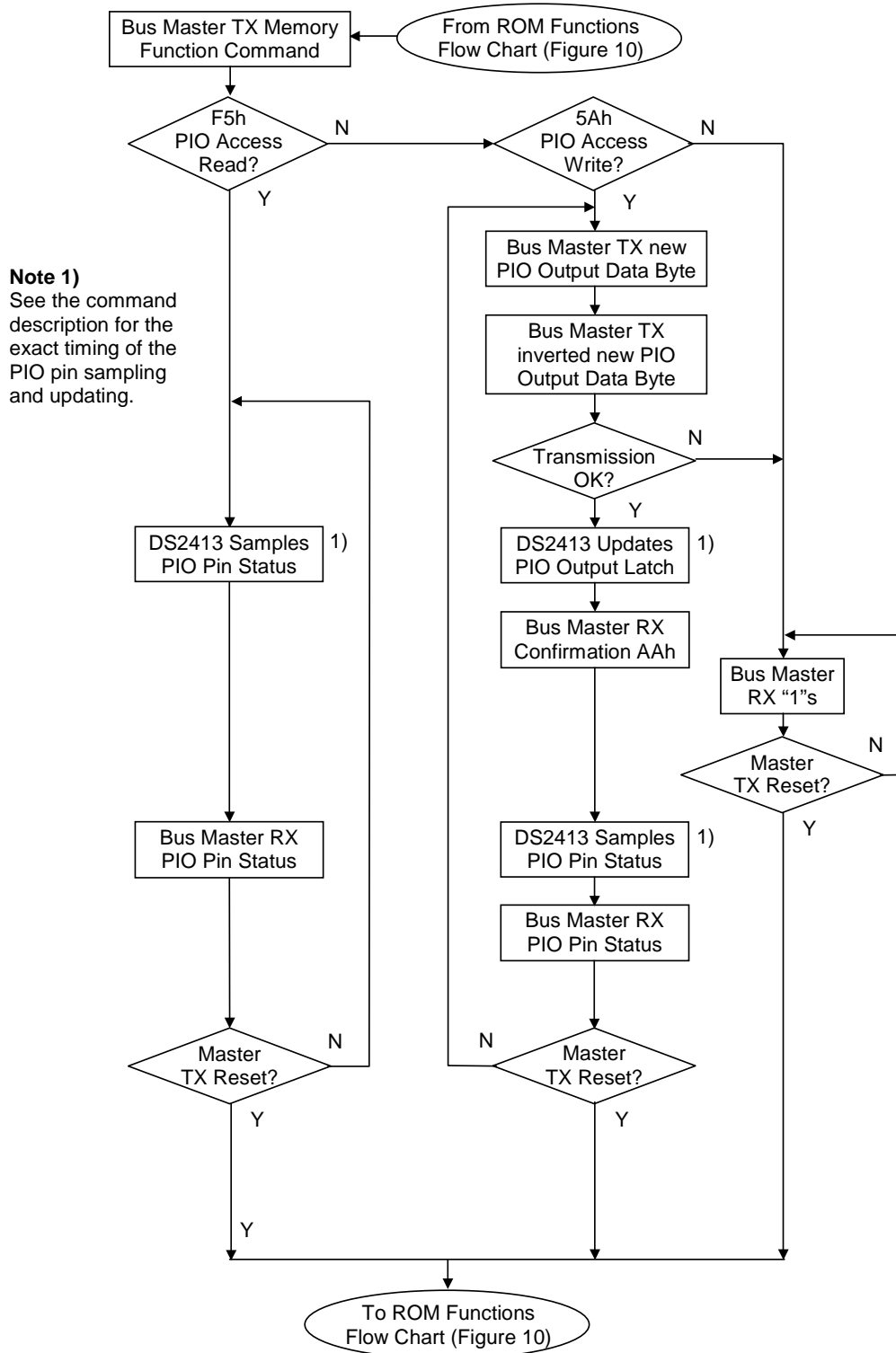
图 6. PIO 功能命令流程图
