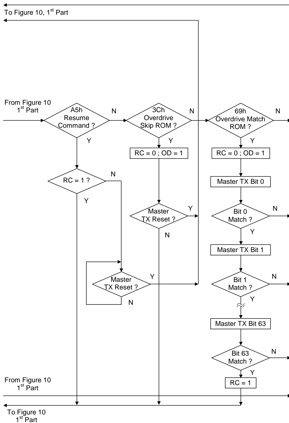
图 10-2. ROM 功能流程图 (续)
