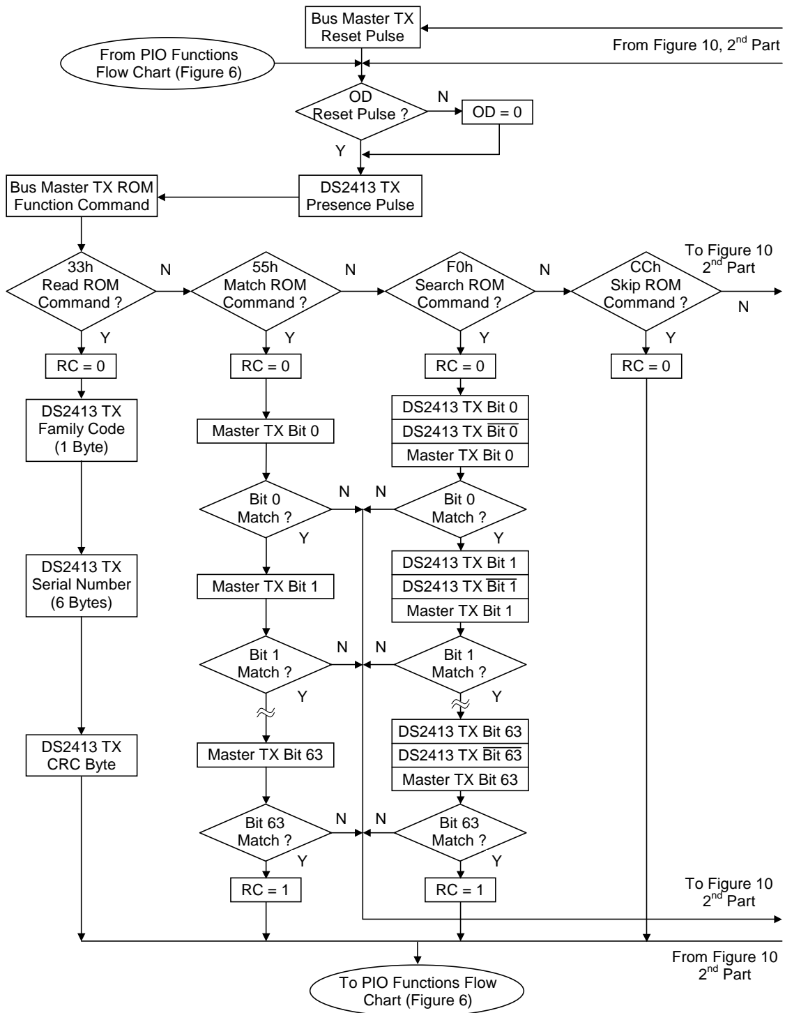
图 10-1. ROM 功能流程图
