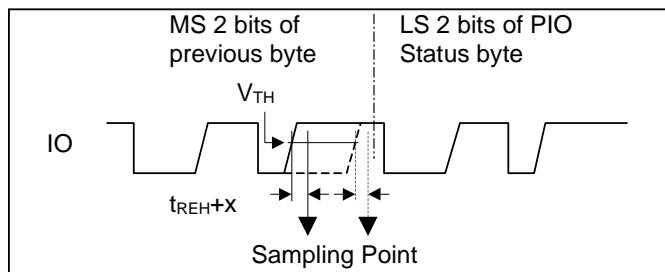
图 7. PIO Access Read 时序图
