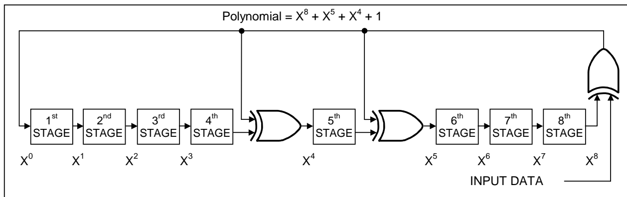
图 4. 1-Wire CRC 发生器
