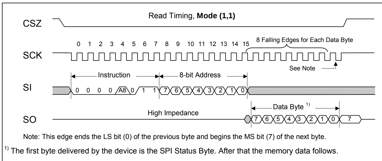
图 20. 读存储器和 PIO 时序 (续)
