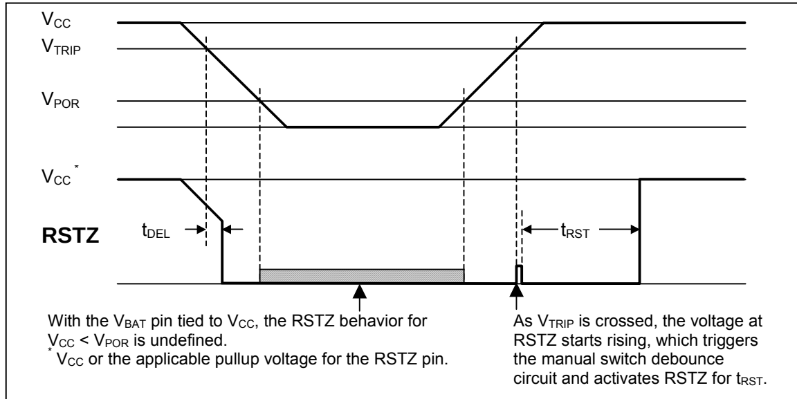
图 6. RSTZ 电源失效复位
