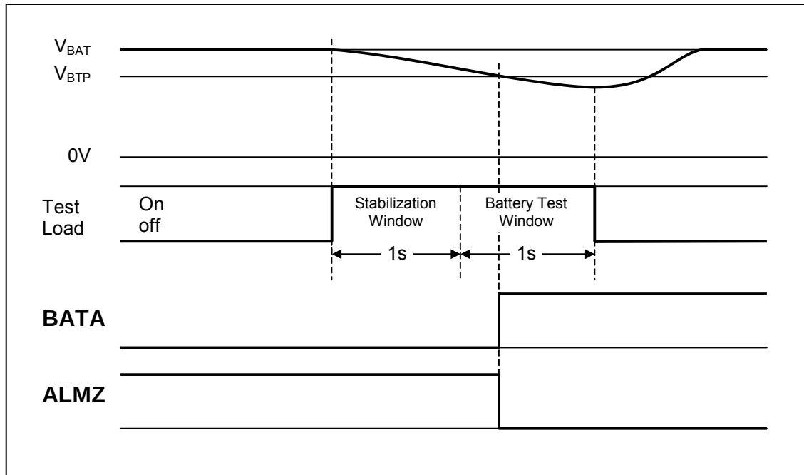
图 8. 电池检测操作
