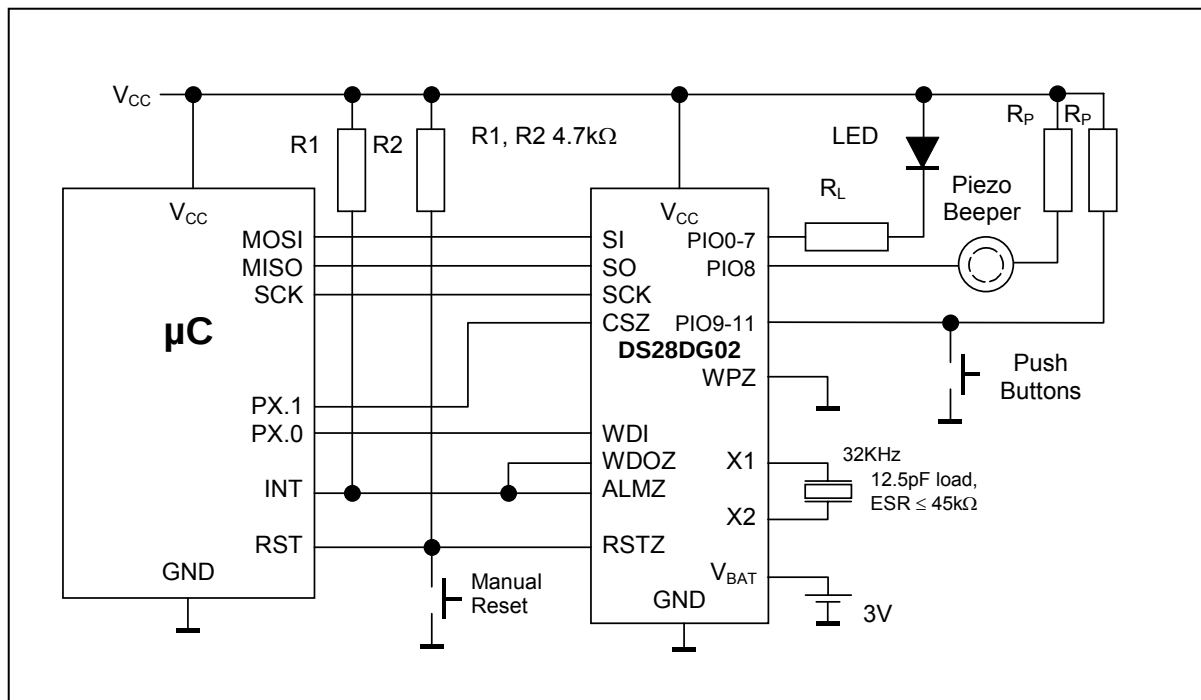
典型工作电路
