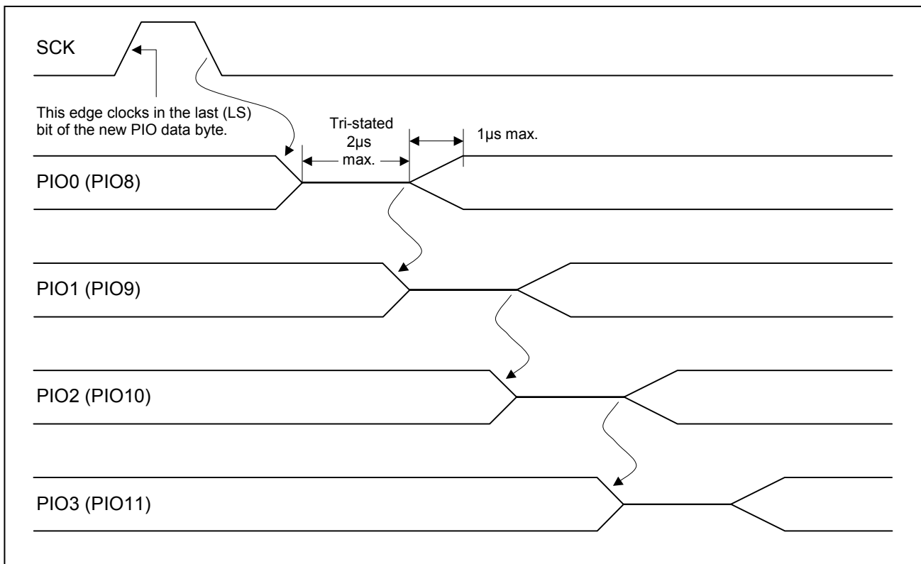
图 22. PIO 写操作时序，大电流模式
