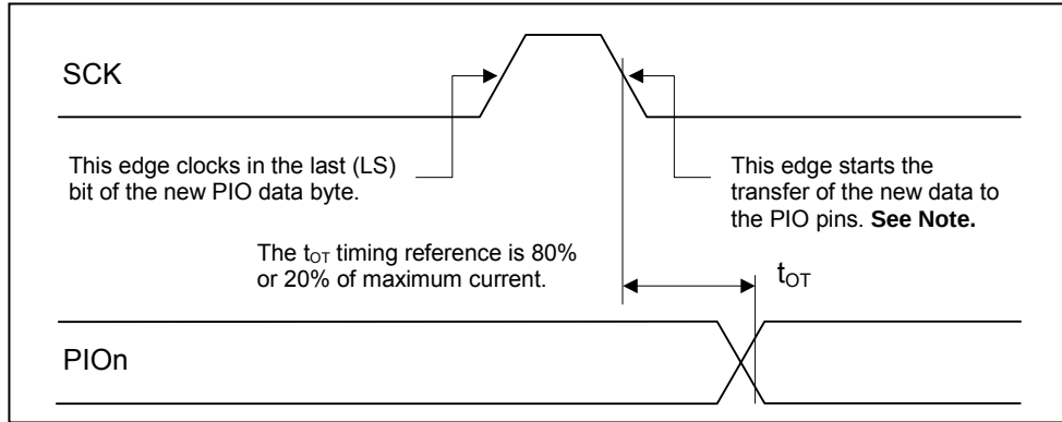
图 21. PIO 写访问时序，小电流模式
