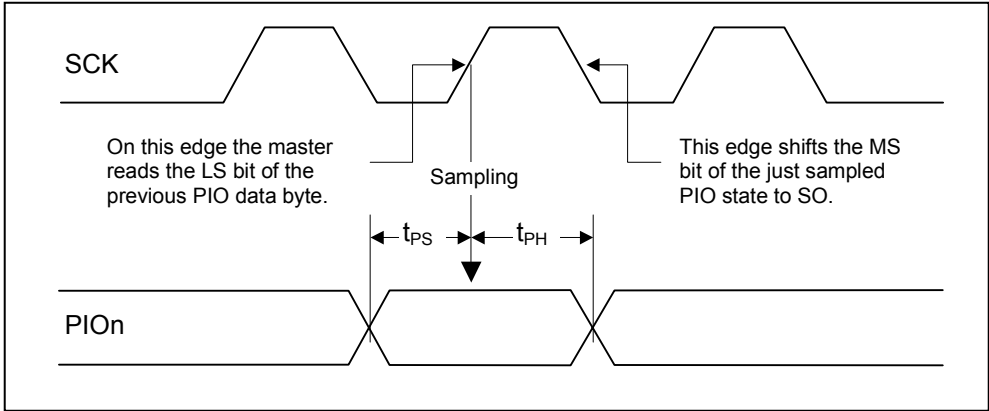
图 23. PIO 读操作时序
