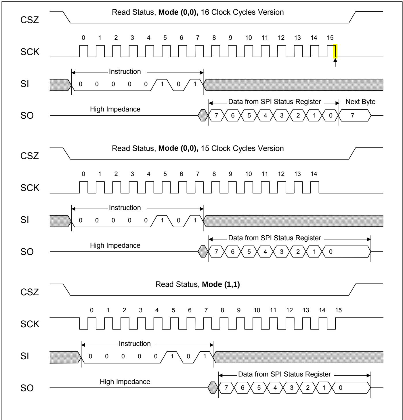
图 16 . 读 SPI 状态寄存器时序
