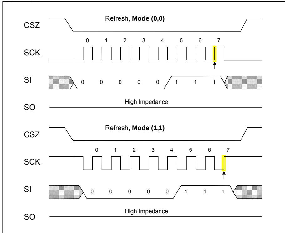
图 17. 刷新 PIO 寄存器时序
