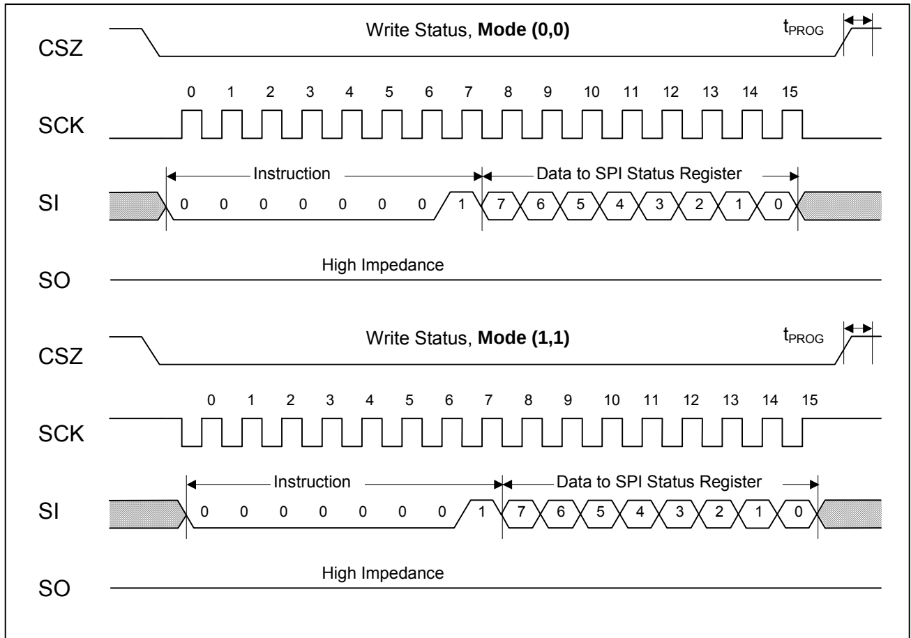
图 15. 写 SPI 状态寄存器时序
