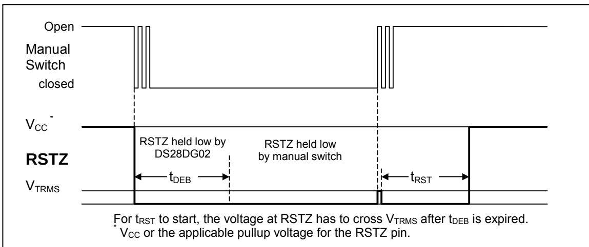
图 7. RSTZ 手动开关去抖
