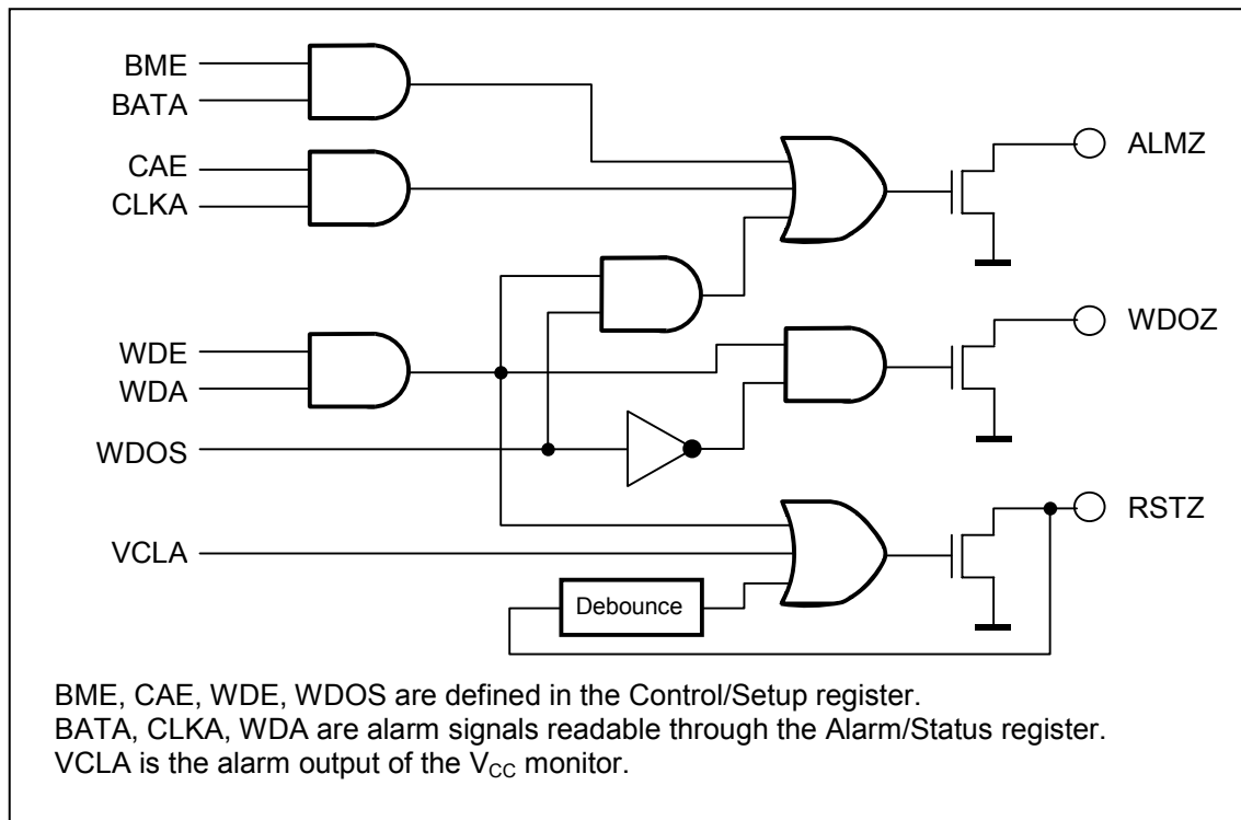
图 5. 产生 ALMZ、WDOZ 和 RSTZ
