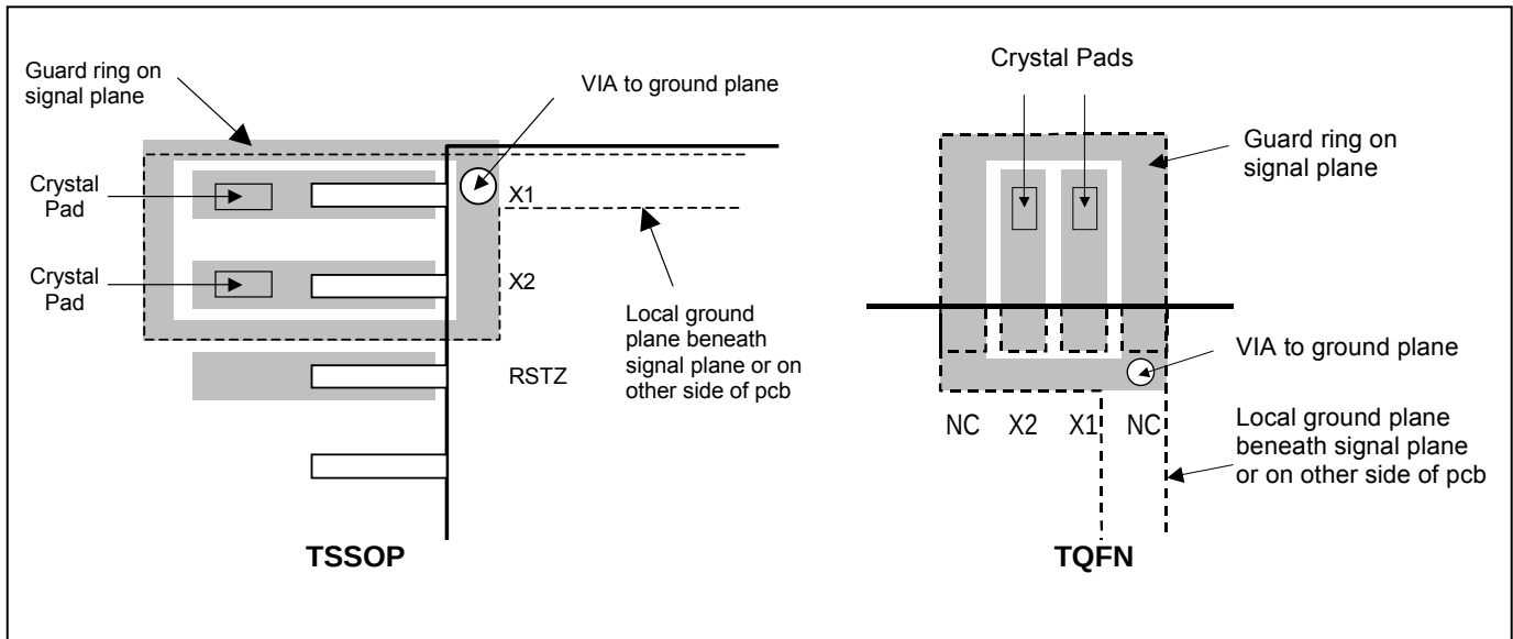
图 24. PCB 中晶体的放置
