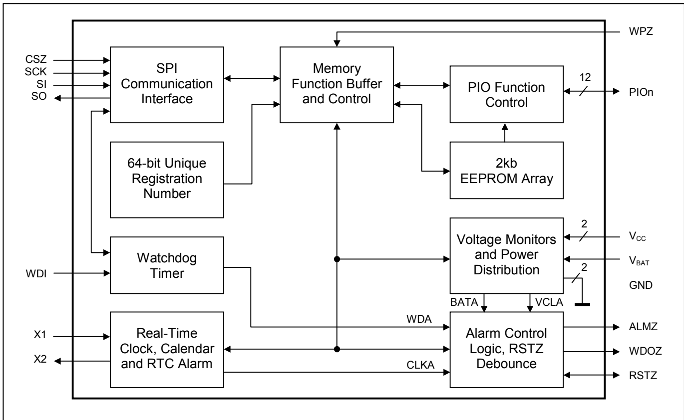
图 1. 功能框图
