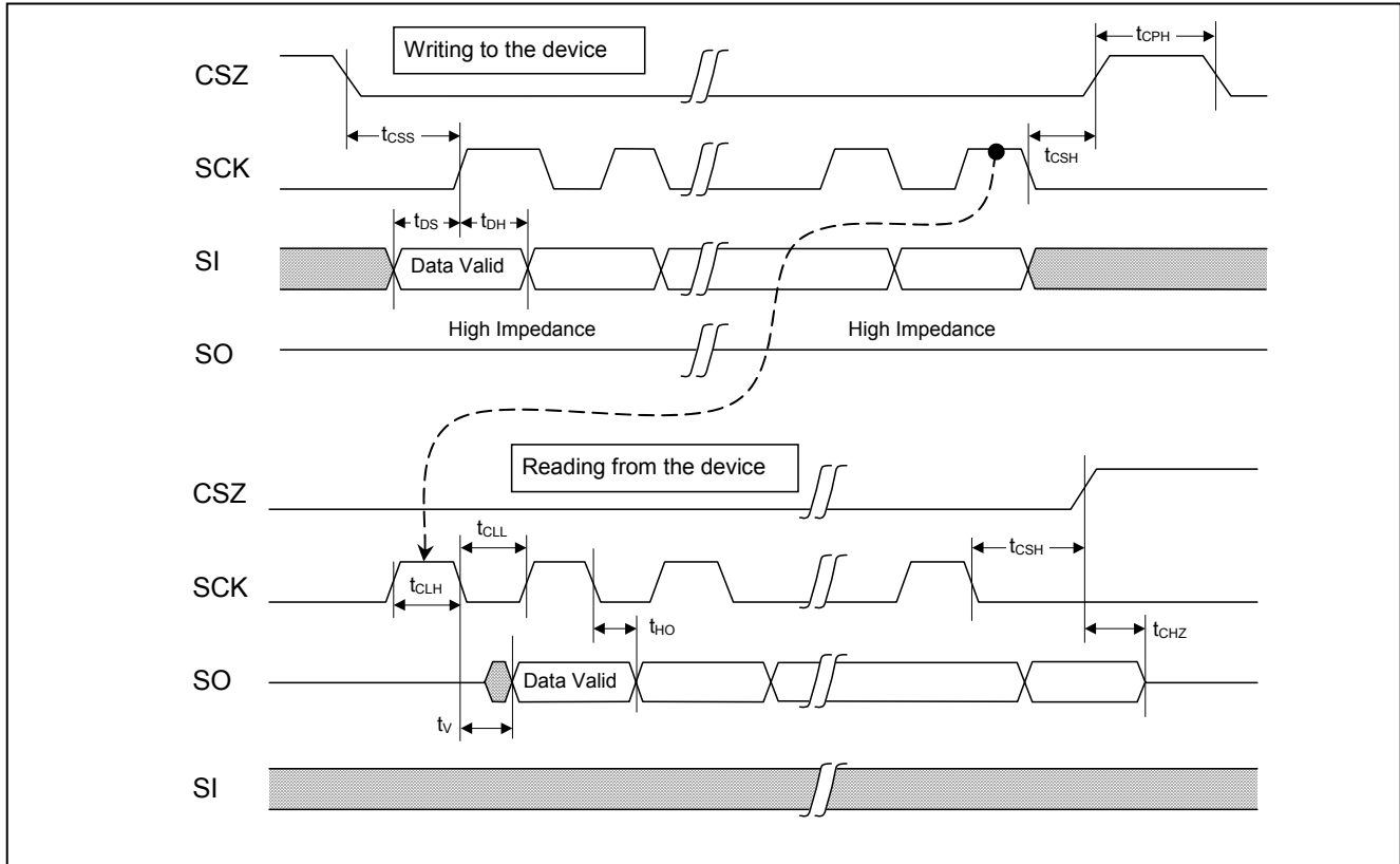
图 9. SPI 时序, 模式(0,0)
