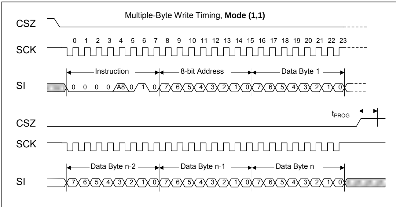
图 19. 存储器和 PIO 的多字节写操作时序 (续)
