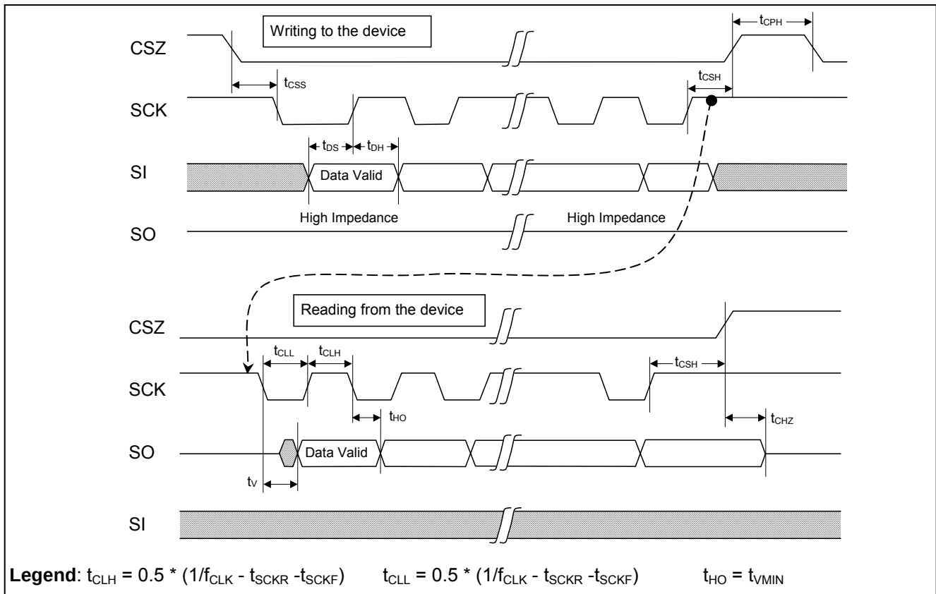
图 10. SPI 时序, 模式(1,1)
