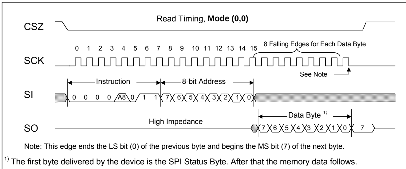
图 20. 读存储器和 PIO 时序
