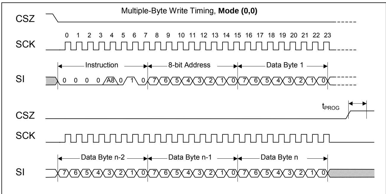
图 19. 存储器和 PIO 的多字节写操作时序
