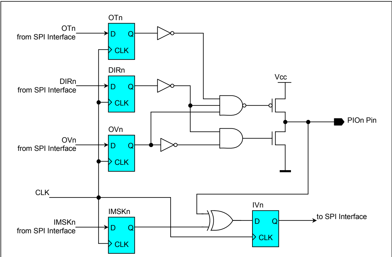
图 4. PIO 简化原理图
