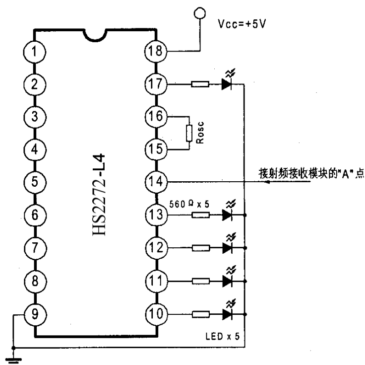
HS2272-L4 (4数据型) 射频应用电路
