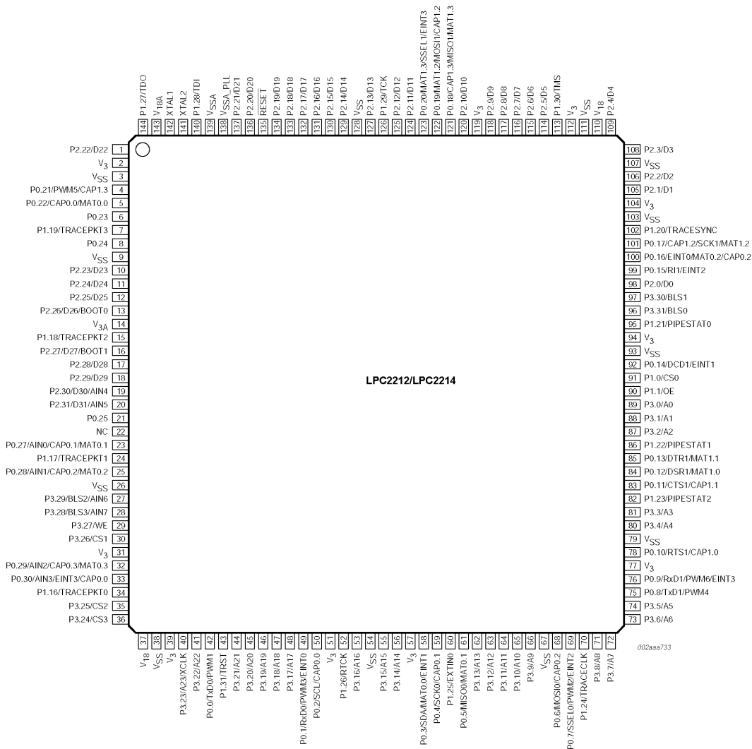
图 2 LQFP144 管脚排列
