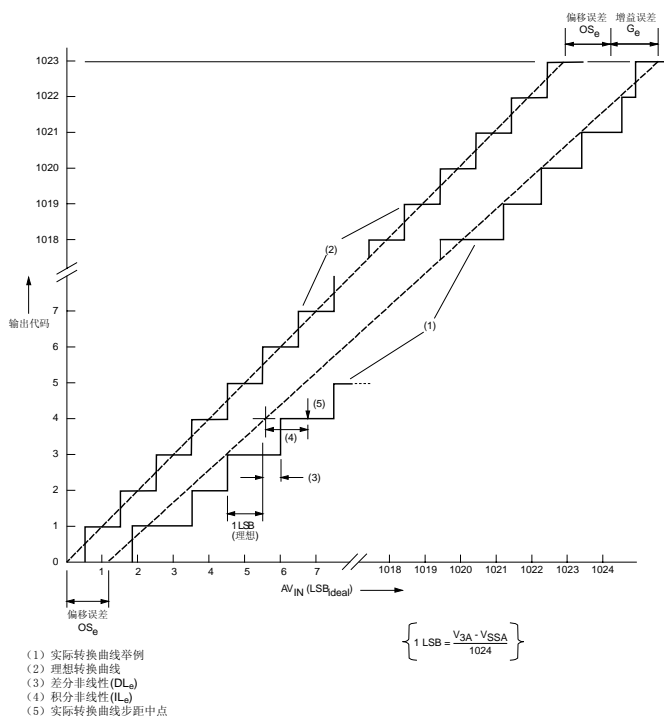
图 4 A/D 转换特性
