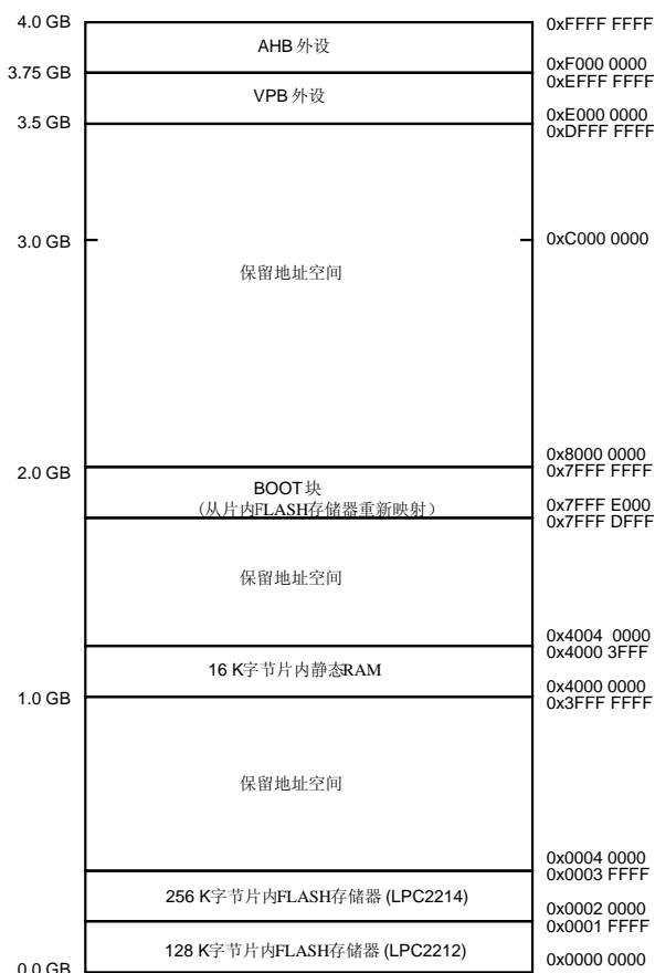
图 3 LPC2212/2214 存储器映射
