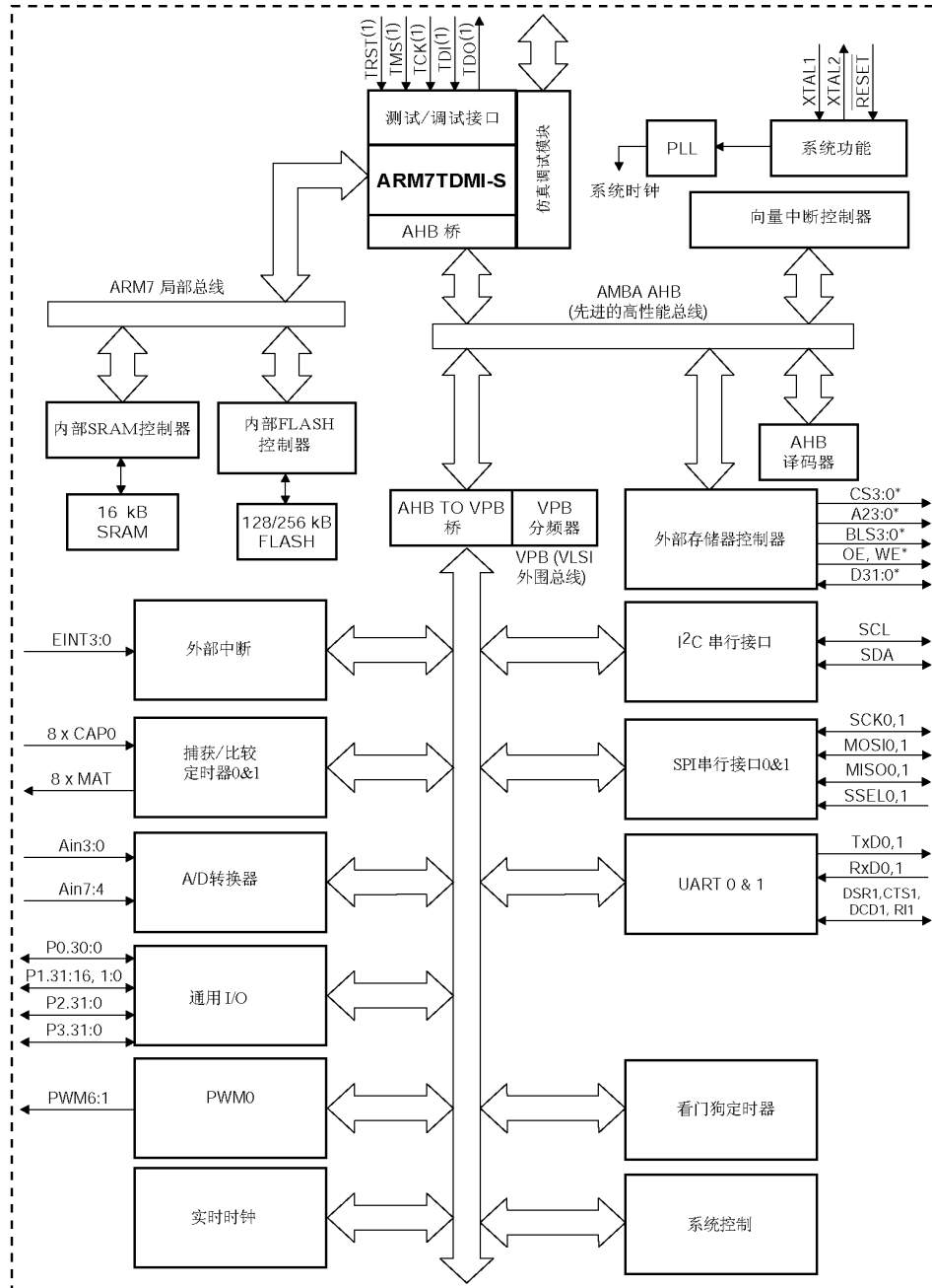
图 1 结构框图
