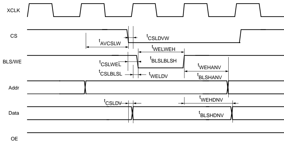
图 6 外部存储器写访问
