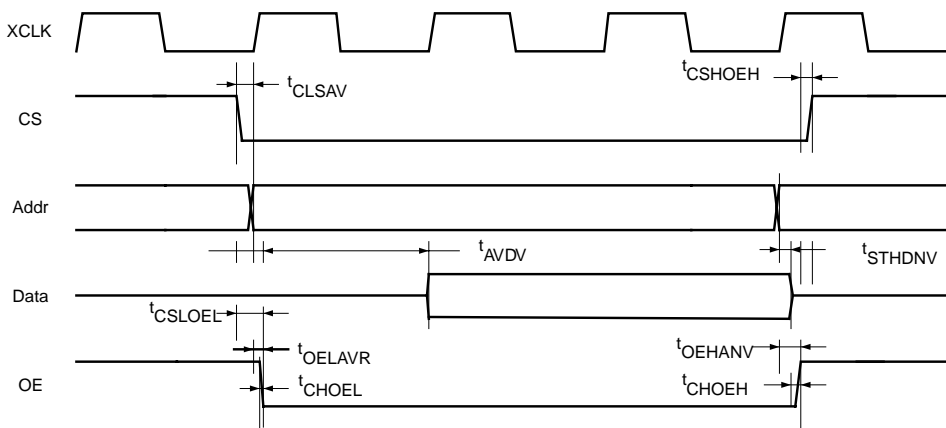
图 5 外部存储器读访问
