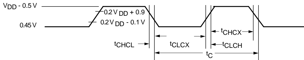
图 7 外部时钟时序
