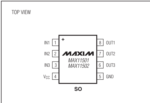
引脚配置
