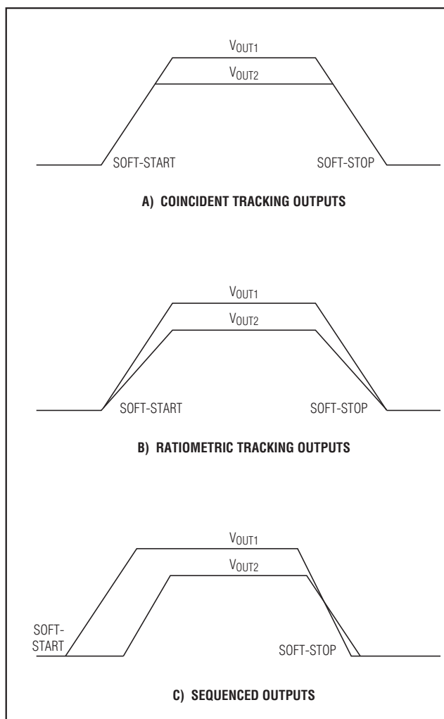
图1. 同步跟踪、比例跟踪和PGOOD排序示意图
