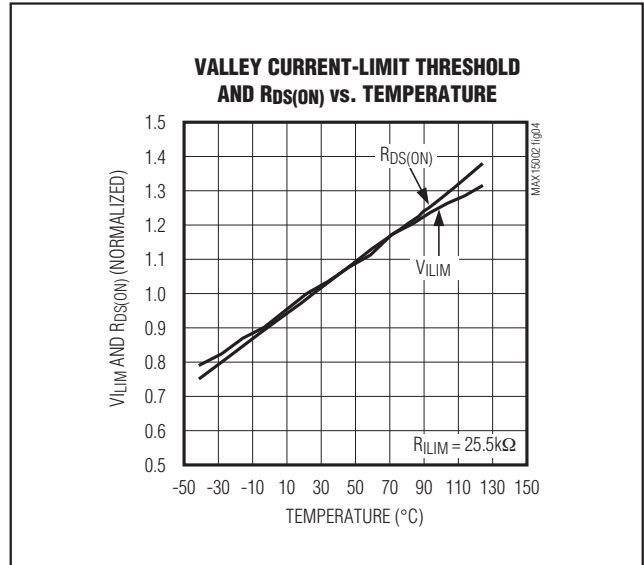
图4. 限流门限点以及 V_{RDS(ON)} 与温度的关系
