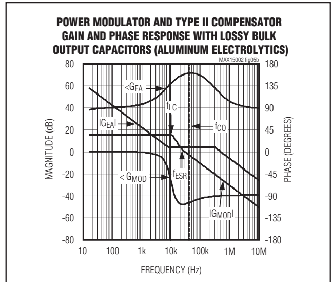
图5b. 电源调制器(较大的 C_{OUT} )和II类补偿器响应
