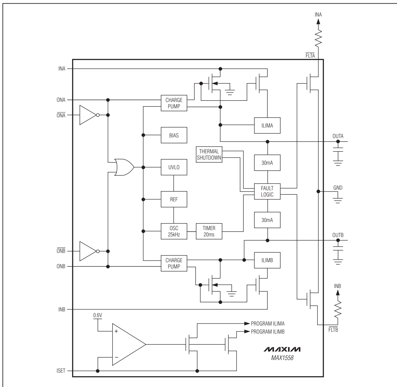
图2. 功能框图
