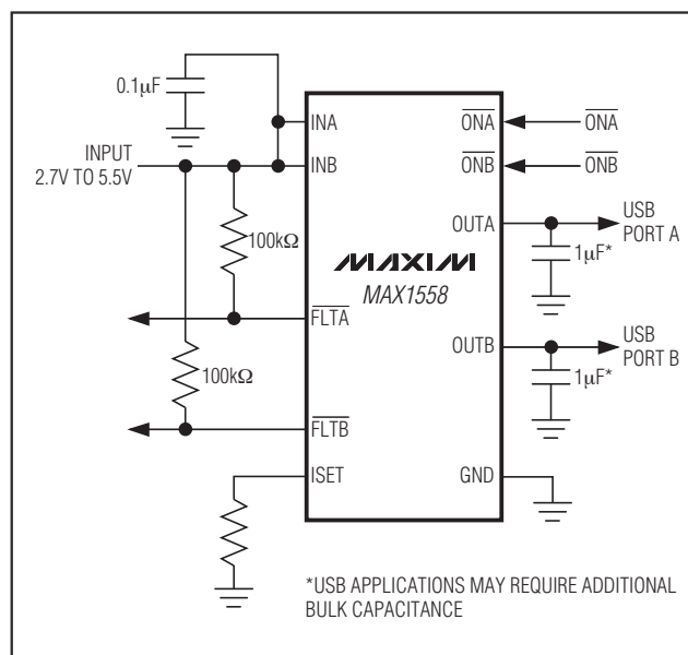
图1. 典型应用电路
