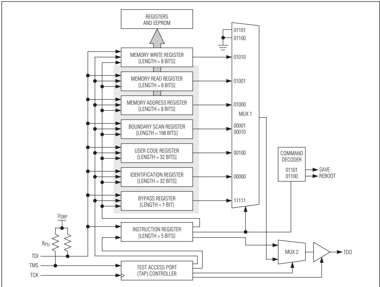
图6. JTAG方框图
