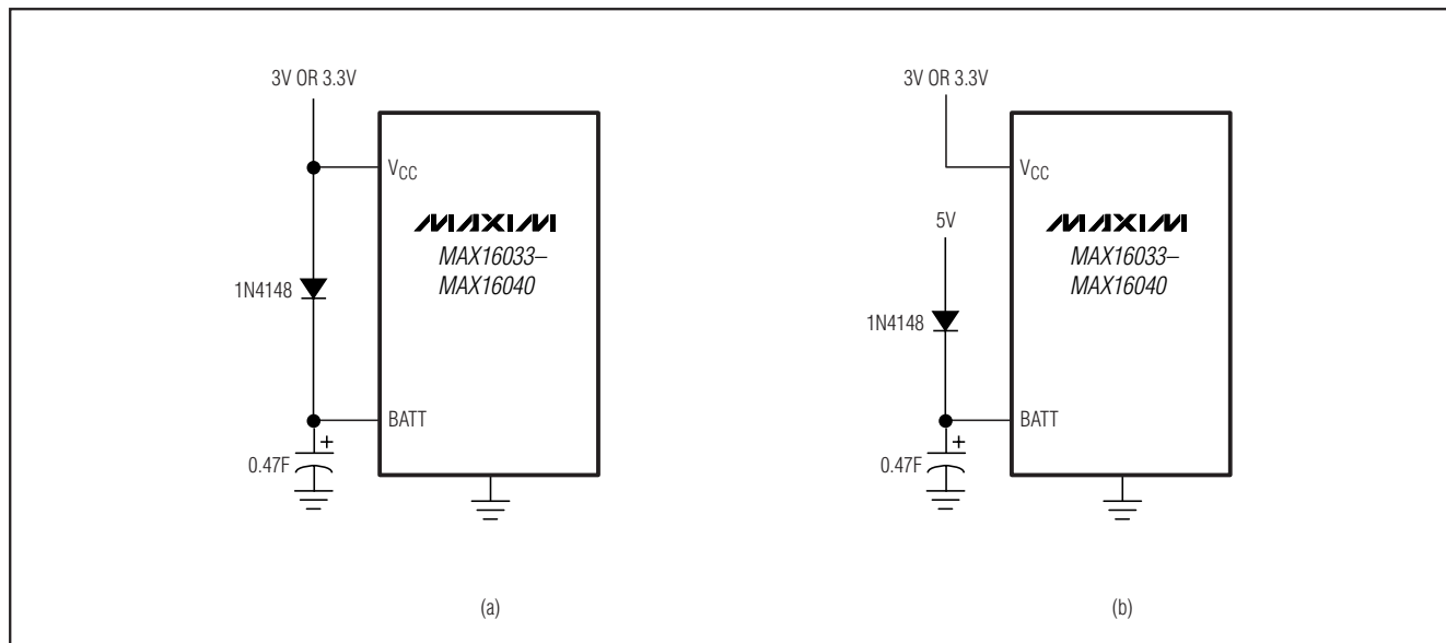
图5. 用超级电容作为备份电源
