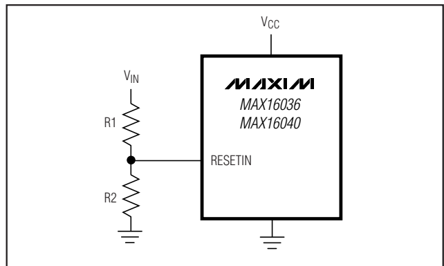
图4. 设置MAX16036/MAX16040的RESETIN电压
