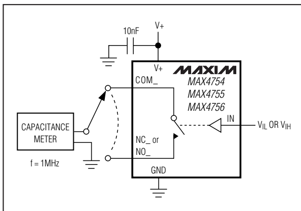
图 5. 通道开/关电容
