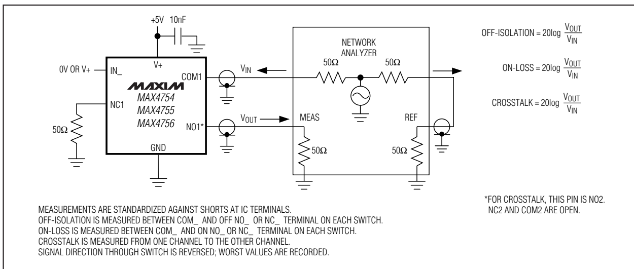
图 4. 导通损耗、关断隔离和串扰
