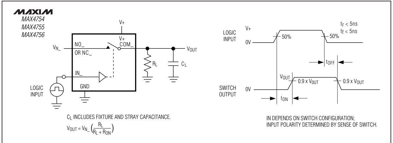
图 1. 开关时间
