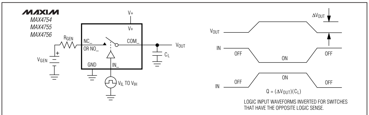
图 3. 电荷注入
