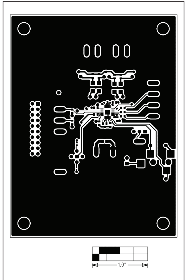
图9. MAX9702评估板PC板布局——元件层
