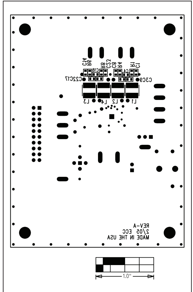
图13. MAX9702评估板元件布局——焊接层
