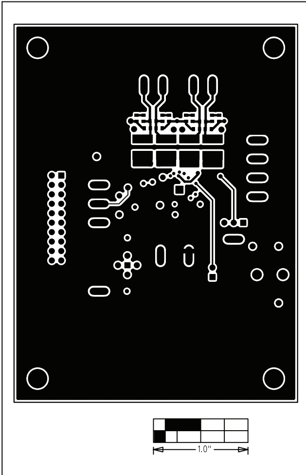
图12. MAX9702评估板PC板布局——焊接层
