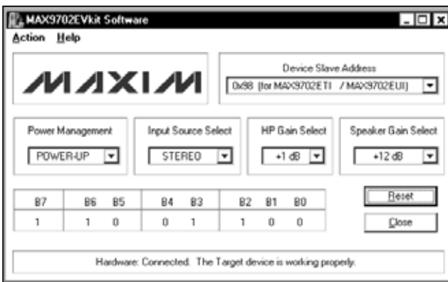
图1. MAX9702评估板软件的主窗口
