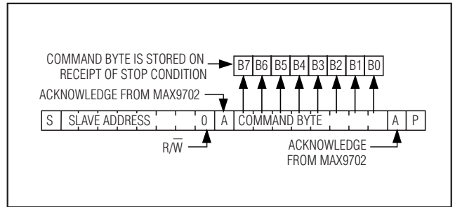
图12. 写数据格式实例
