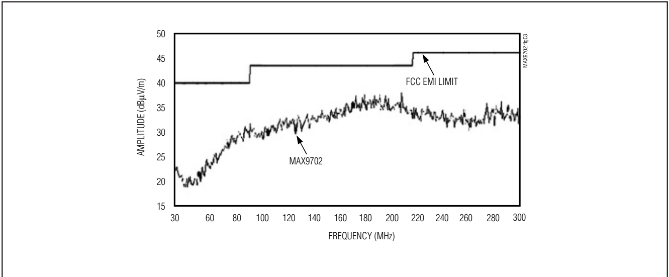
图3. 采用76mm扬声器电缆时, MAX9702的EMI
