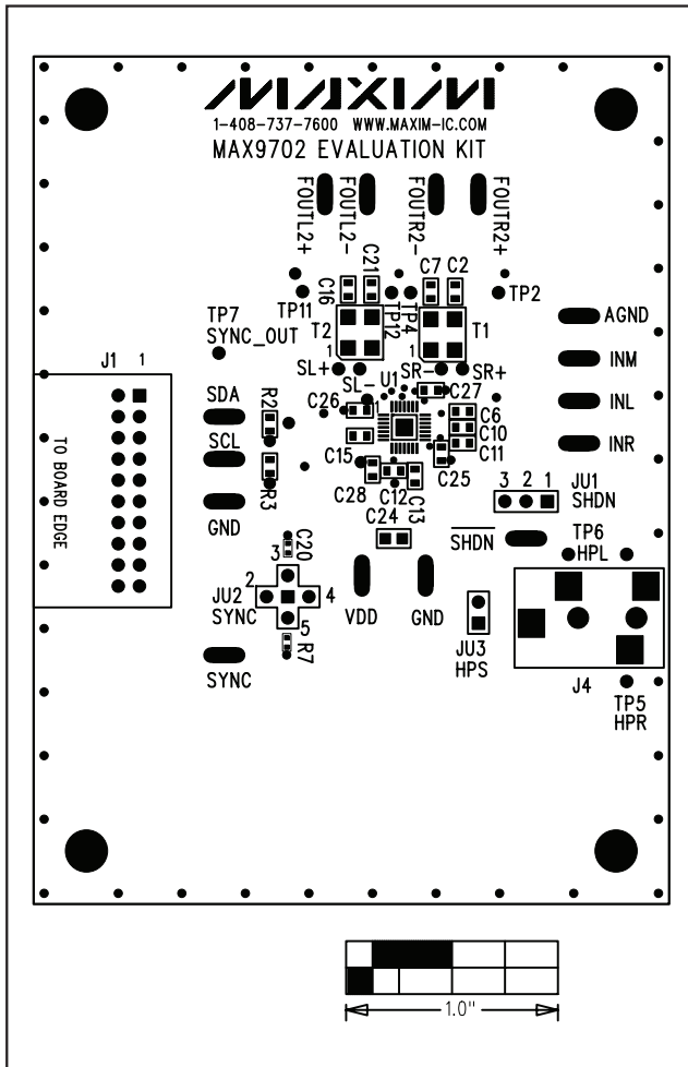
图8. MAX9702评估板元件布局——元件层
