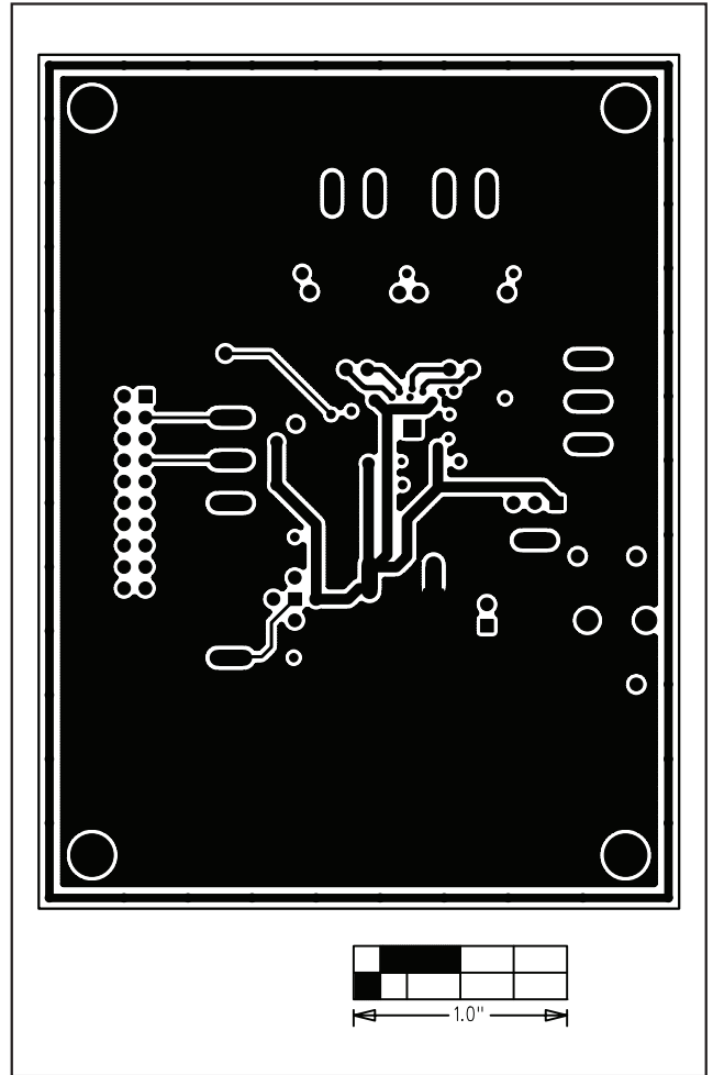
图11. MAX9702评估板PC板布局——第3层 (电源)
