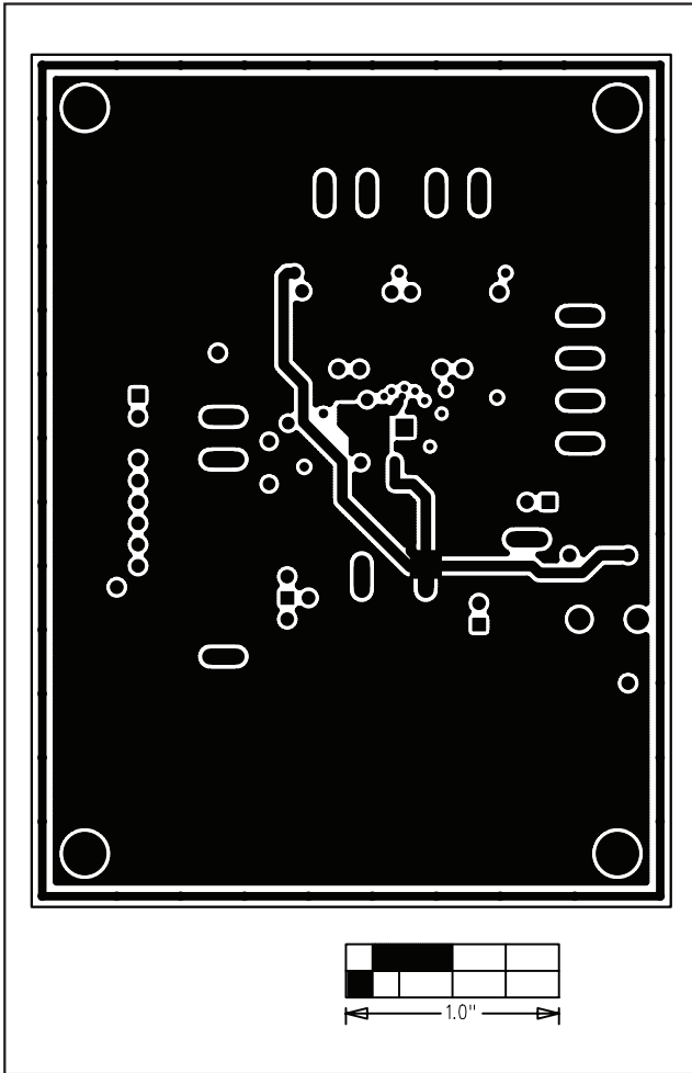
图10. MAX9702评估板PC板布局——第2层 (地)
