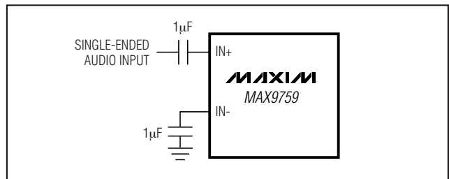
图6. 单端输入
