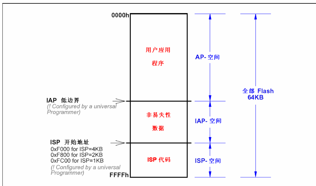
图 20-1. Flash 结构
