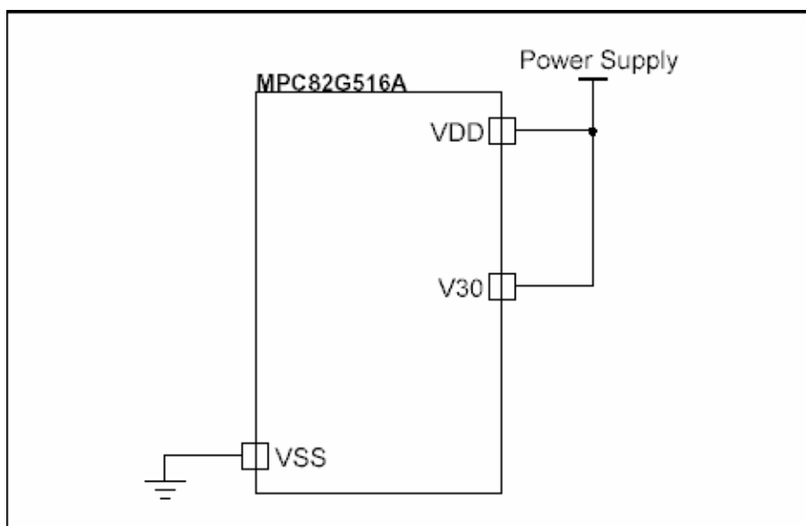
图27-2. 3.3V 供电
