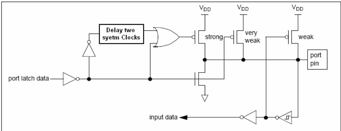
图 10-1 准双向 I/O
