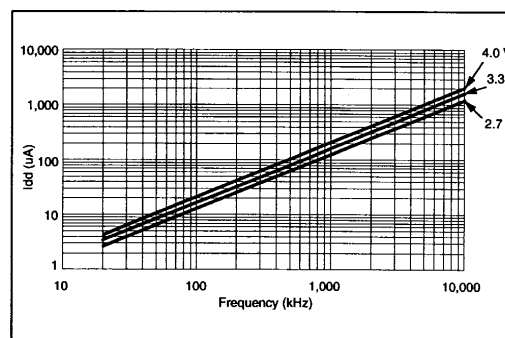
图 44 典型的空闲 Idd 对应频率(外部时钟, 25°C, LPEP=1)
