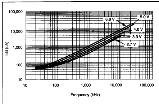
图 45 典型的使用中 I_{dd} 与对应频率 (外部时钟, 25°C, LPEP=0)
