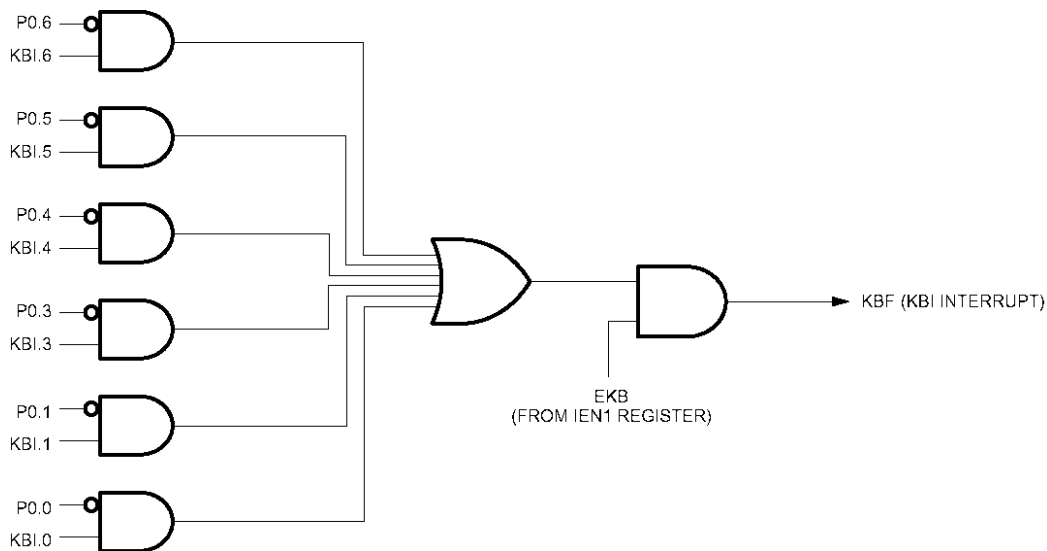
图 13 键盘中断
