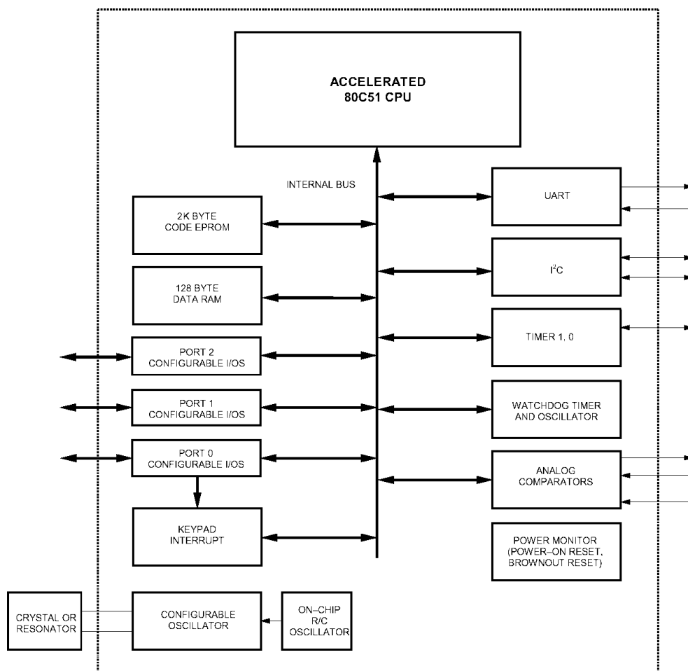
功能框图
