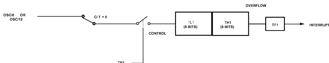
图 25 模式 1 时定时器 1 (16 位定时器)
