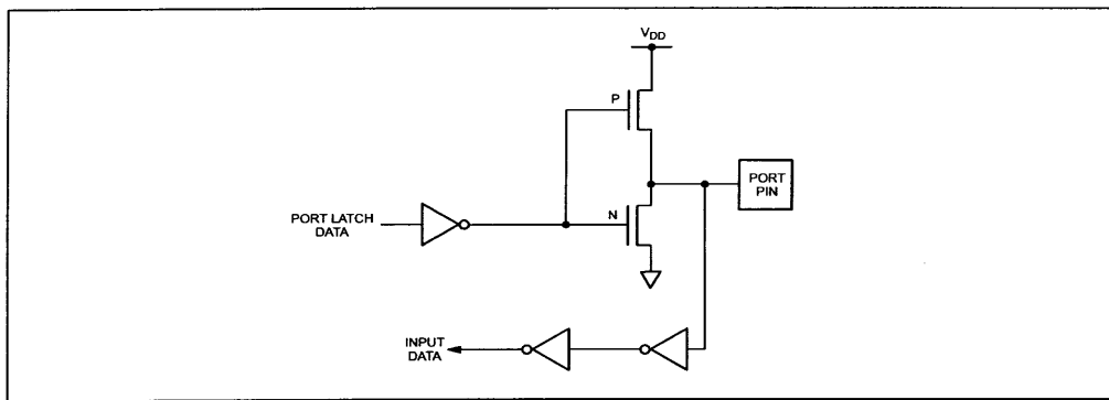
图 11 上拉输出
