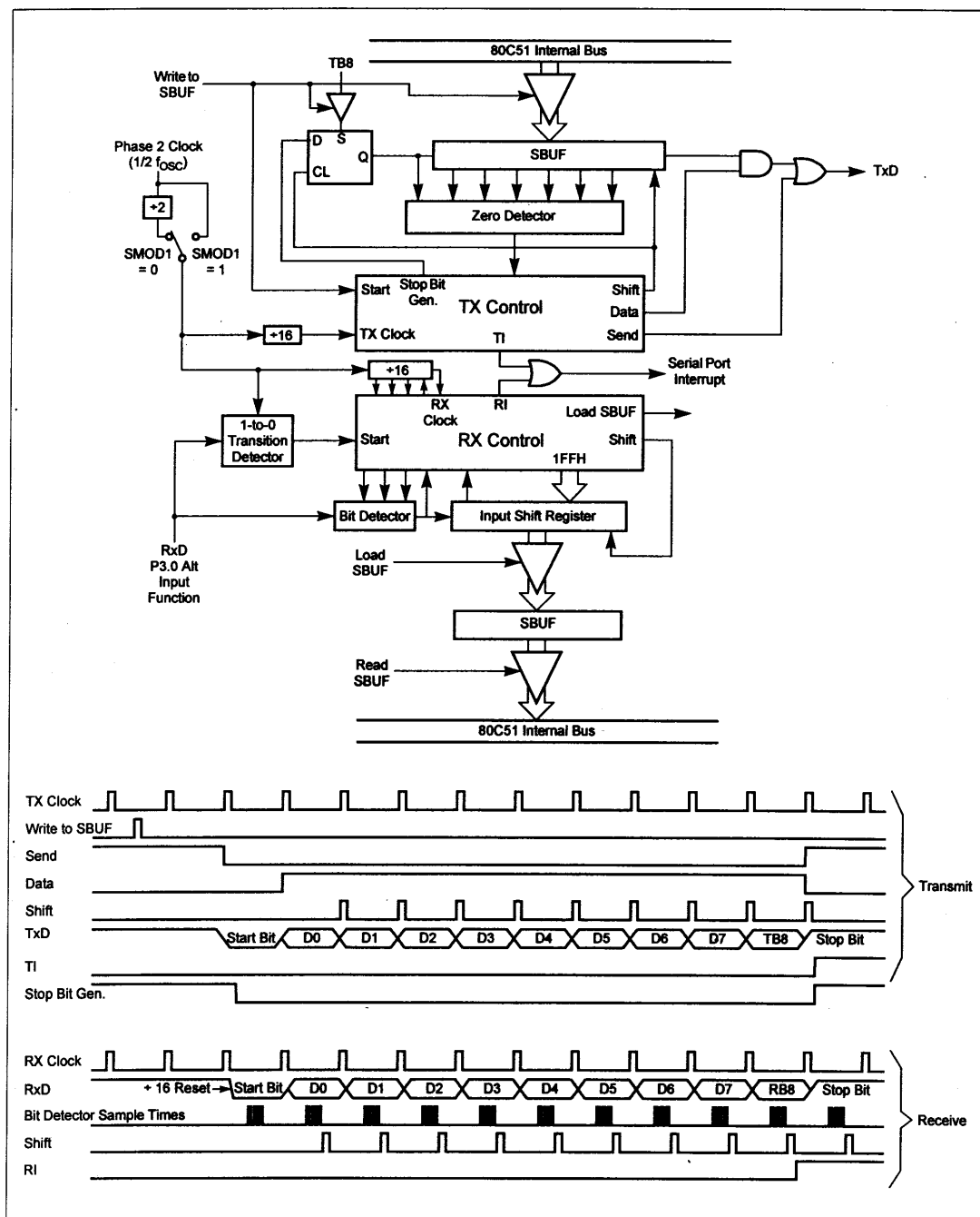
图 32 串口模式 2
