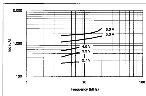
图 43 典型的高频振荡器 Idd(25°C)
