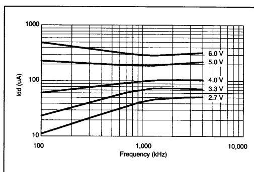
图 42 典型的中频振荡器 Idd(25°C)
