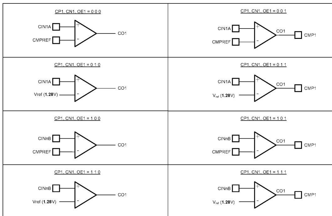
图4 比较器配置
