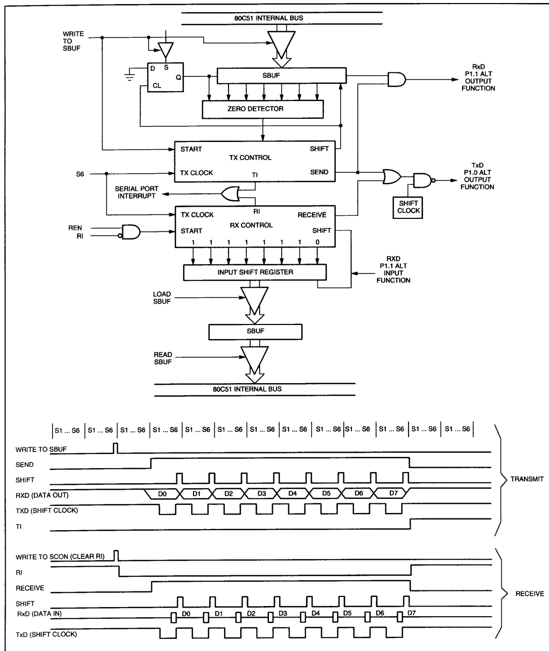
图 30 串口模式 0
