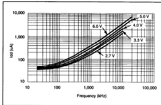
图 46 典型的空闲中 I_{dd} 与对应频率(外 部时钟, 25°C, LPEP=0)
