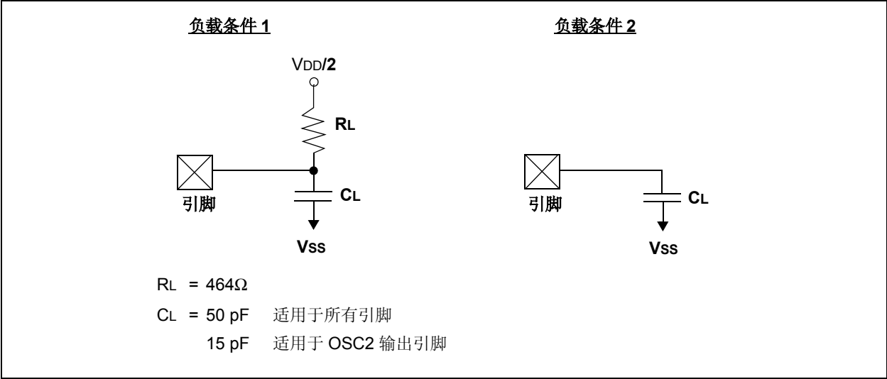
图 12-4: 负载条件
