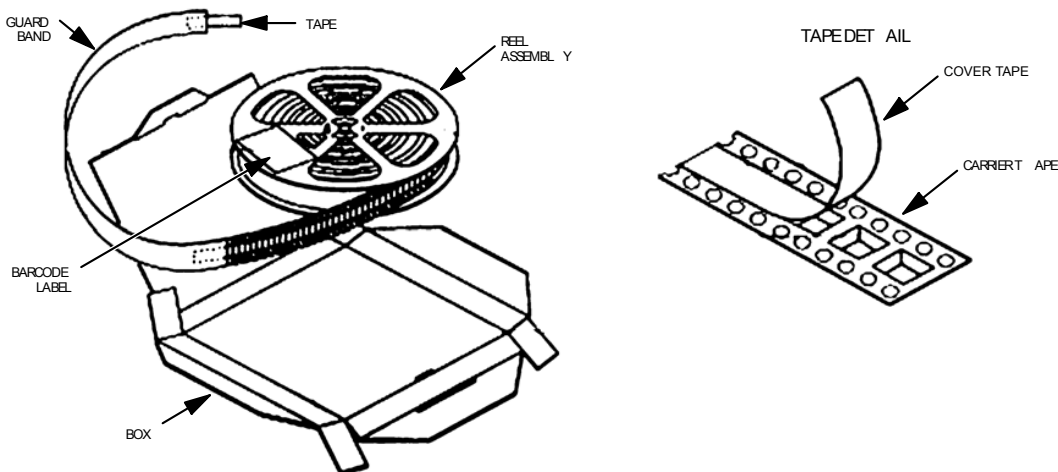
图 4 磁带和卷盘封装方式
