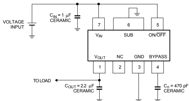
图 3 典型的应用电路
