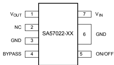
图 2 管脚配置
