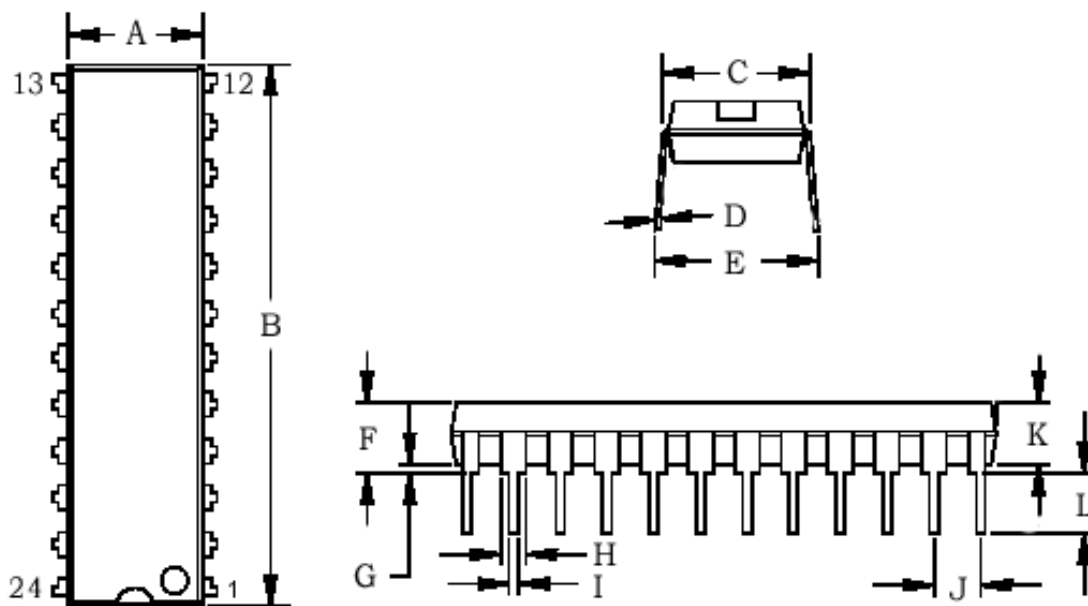
DIP 封装尺寸图 图 10
