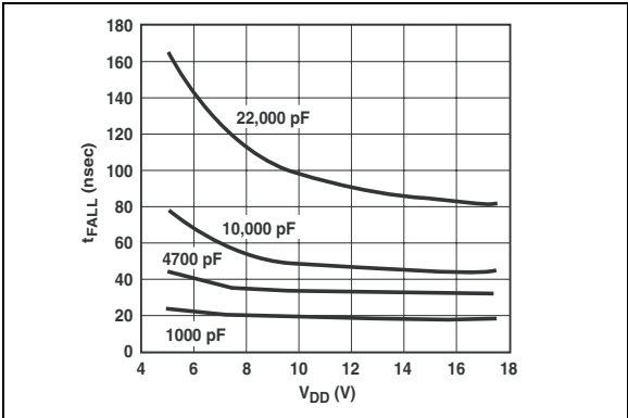
图 2-4: 下降时间—供电电压曲线
