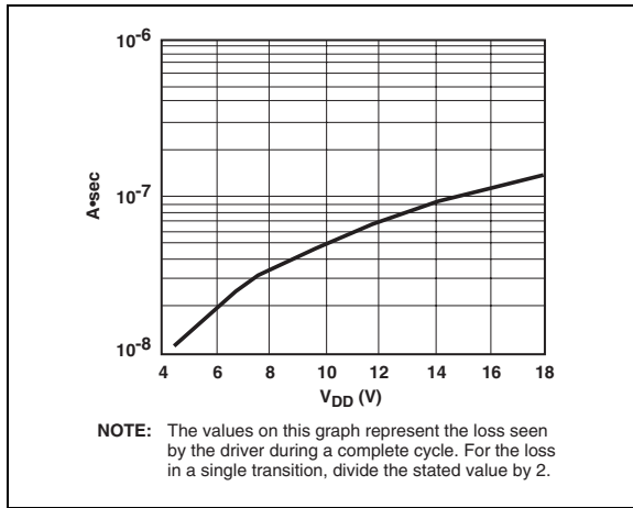
图 2-14: 交叉能量—供电电压曲线
