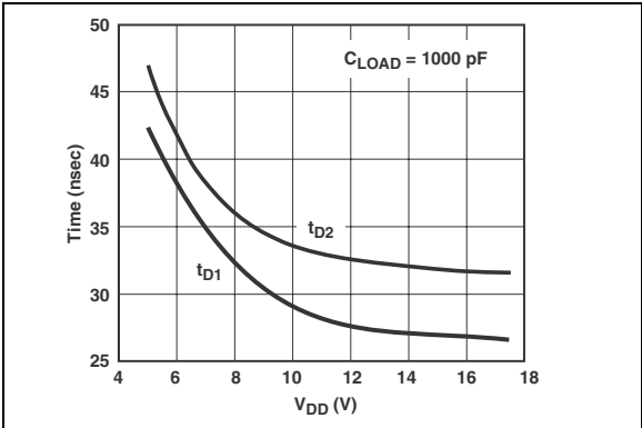
图 2-6: 传播延时—供电电压曲线
