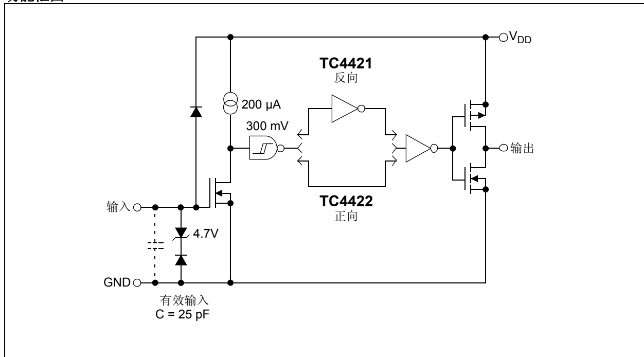
功能框图
