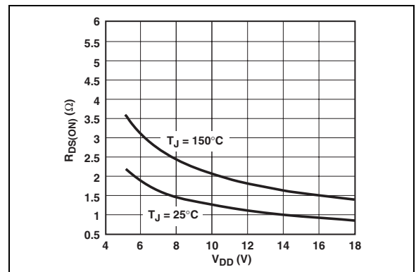
图 2-18: 低阻态输出阻抗—供电电压曲线
