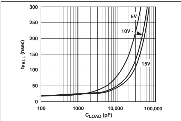
图 2-5: 下降时间—容性负载曲线
