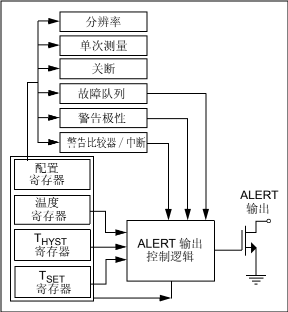
图 4-2: 寄存器框图
