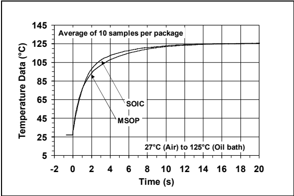
图 2-9: TCN75A 热响应——时间曲线
