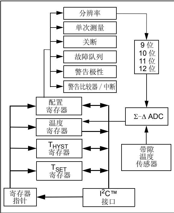
图 4-1: 功能结构框图
