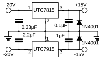
图11 分电源电路( \pm 15\text{V} , 1\text{A} )
