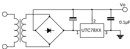
图10 跟踪电压稳压电路
