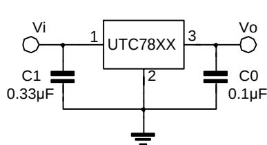
测试电路图
