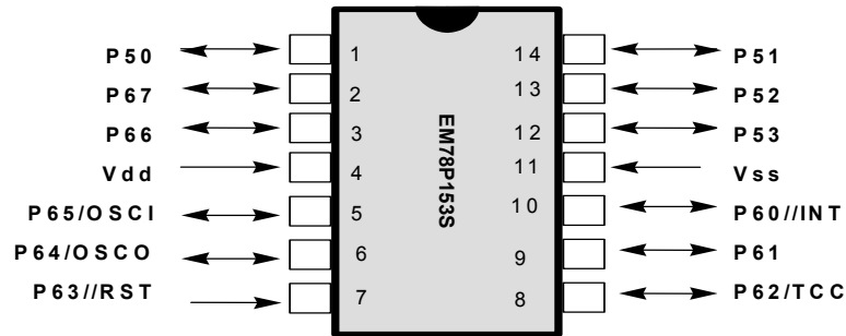
图1 管脚分配
