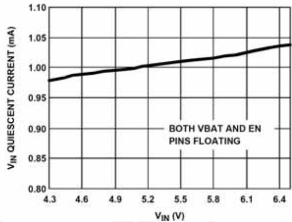
图 14 输入静态电流与输入电压的关系（不关断时）
