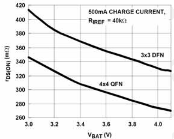
图 10 r DS(ON) 与输出电压的关系（使用限定电流的适配器时）
