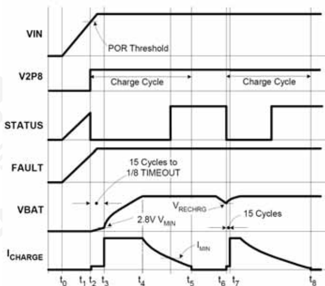
图 19 工作波形图
