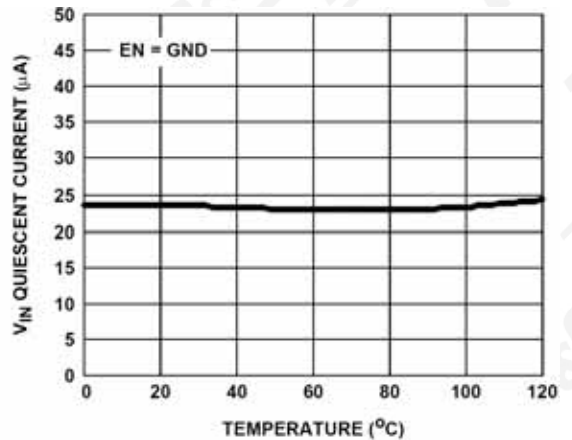
图 12 输入静态电流与温度的关系
