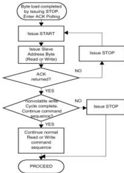
图 9 应答查询序列
