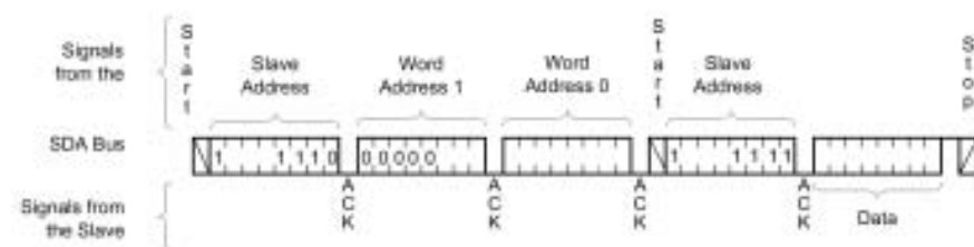
图 10 随机地址读序列
