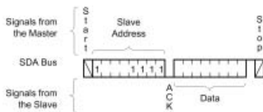
图 8 当前地址读序列
