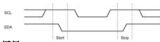
图 4 有效的“开始”和“停止”条件
