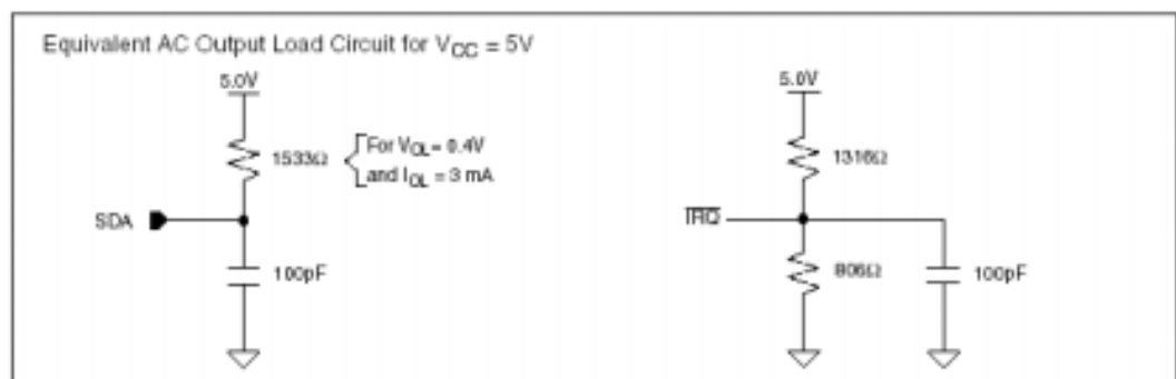
图 14. V_{CC}=5.0V , 测试器件时的标准输出负载
