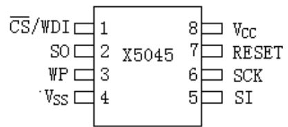
8引脚PDIP/SOIP/MSOP封装
