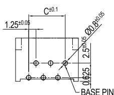
P.C.B. LAY-OUT(A-TYPE)
