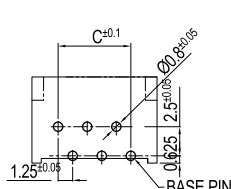
P.C.B. LAY-OUT(B-TYPE)
