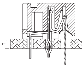
PCB ASS'Y
