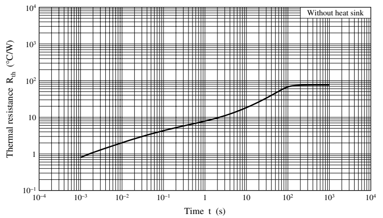
R_{th} - t
