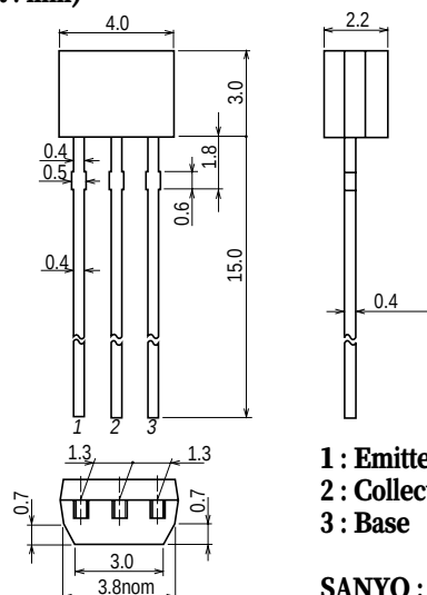
外形図 2033A (unit : mm)
