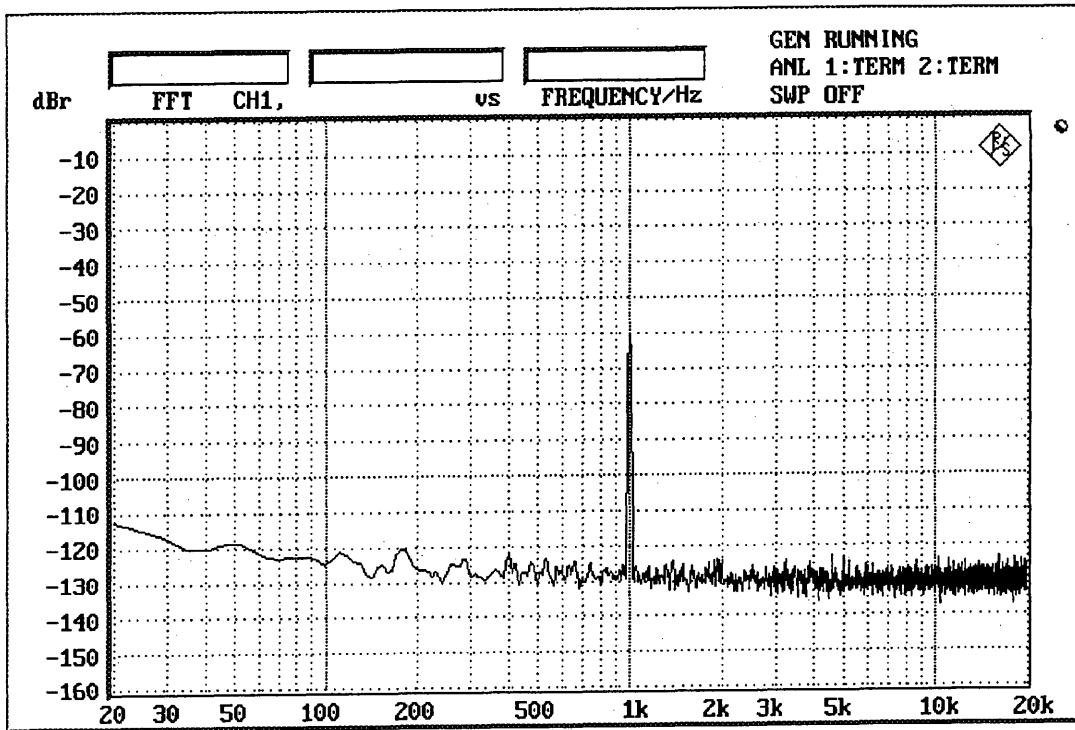
Figure 50 : FFT (input signal : 1kHz, -60dBFS ;
