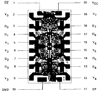
DIE SIZE 0.077" X 0.047"
