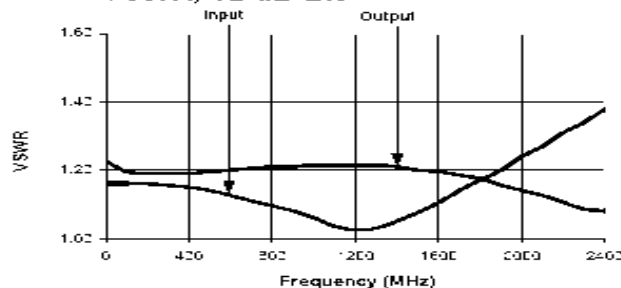
VSWR, 32 dB Bit
