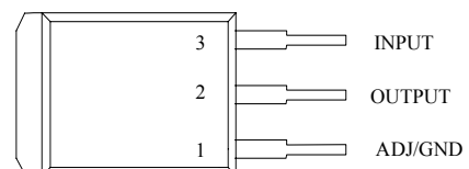
TO-263-3L
