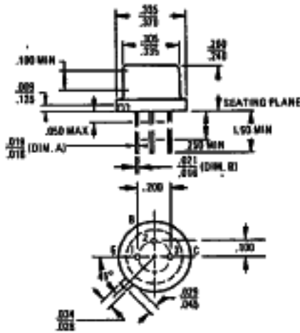
TO-5
