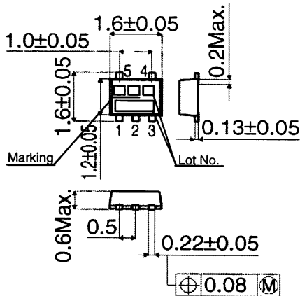
VSO5F5 (UNIT:mm)
