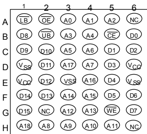
48-Ball CSP top View
