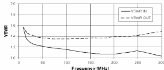
VSWR
