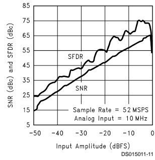
SNR and SFDR vs Input Amplitude
