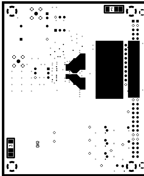
CLC730079 Layer 3
